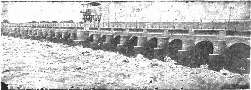
سد الهندية الذي أنشئ شمالى مدينتى الحلة وكربلاء لرى الأراضي جنوبى العراق
