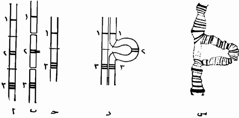
(شكل ٧٨) نقص متباين الازدواج فى كروموسومات الغدة اللعابية . ١ - أشكال تخطيطية ، (س) العينة الفعلية . (عن : ألتبرج ١٩٥٧)
