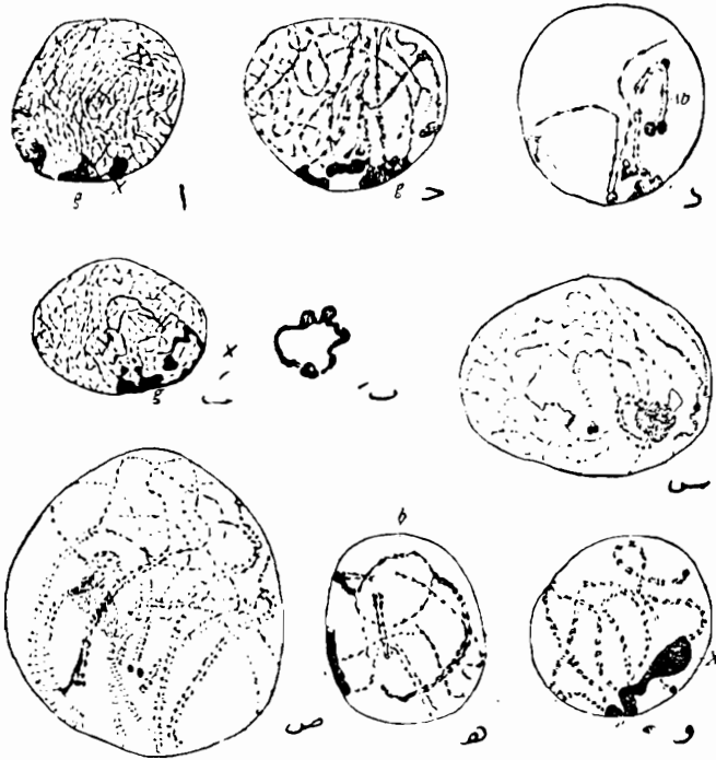
(شكل ٧٦) المرحلة التحضيرية للانقسام الاختزالي الأول في حشرات النطاط ، وهو يبين النمط المنتظم للكروموسومات ، ونوعية الاعتناق . (عن : ويلسون ١٩٢٥) .
