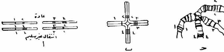
(شكل ٨٠) حالة انتقال غير سليم متباين الازدواج ١. أ، ب : أشكال تخطيطية ، ح : الكروموسومات الفعلية . (عن : ألتبرج ١٩٥٧)
