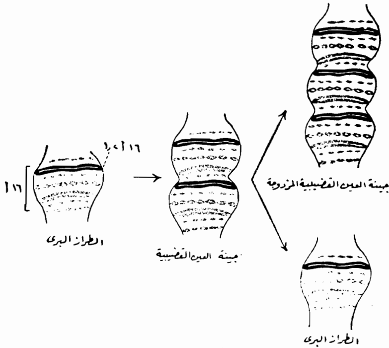
( شكل ٨١ ) « جينة » الخالة القضيبيية في كروموسومات الغدة المعابية « للدرسوفلا » . ( عن : بريدجز وساتون من هوايت ١٩٥٤ )
