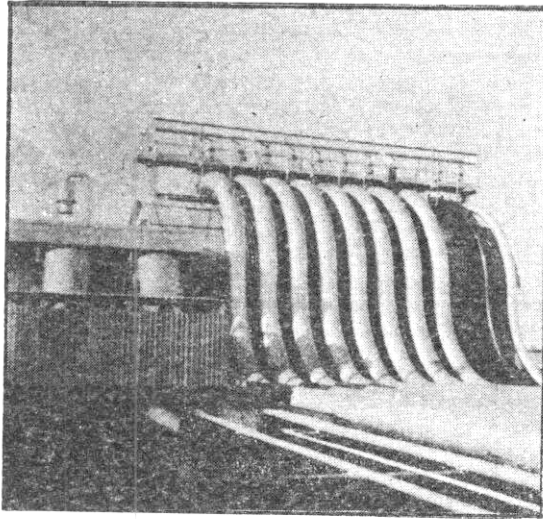
منظر لأتابيب الزيت على أسكلة ميناء الأحمدي
