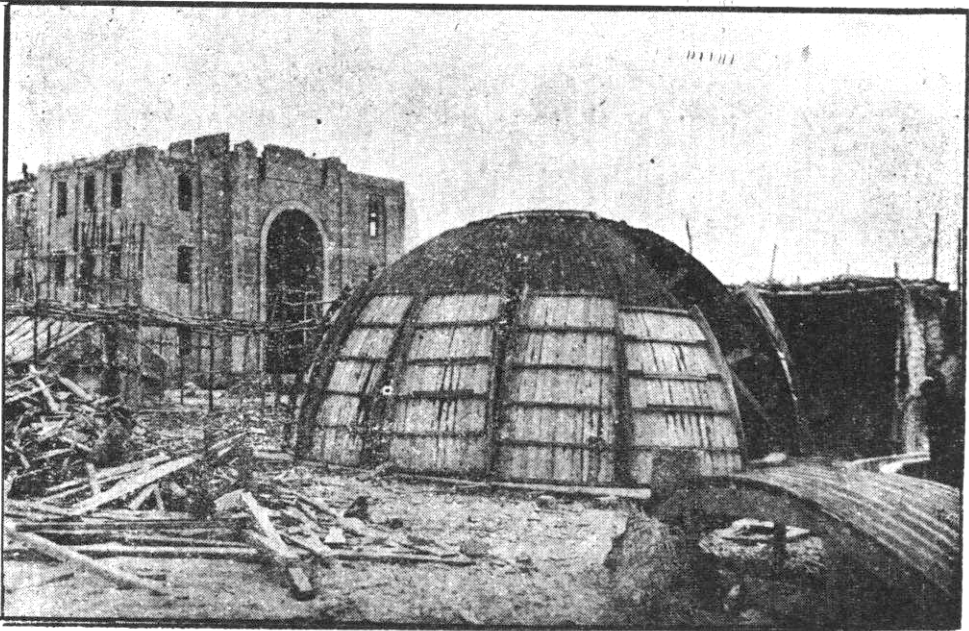
يجرى العمل بهم ونشاط لإنهاء المدرسة الثانوية الداخلي الكبرى في الكويت وهذه الصورة تمشا منظر القالب الخشب لقبة المدرسة في الشوي
