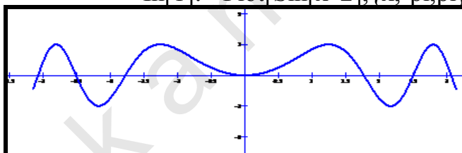
شكل (١٠) الرسم البياني لدالة \text{Sin}(x^2)
