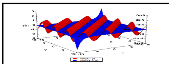
شكل (١١): الرسم البياني للدالتان \text{Sin}[x-y] , \text{Sinh}[x+y]
