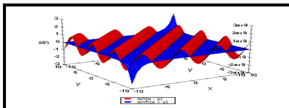
شكل (11): الرسم البياني للدالتان \text{Sin}[x-y] , \text{Sinh}[x+y]
