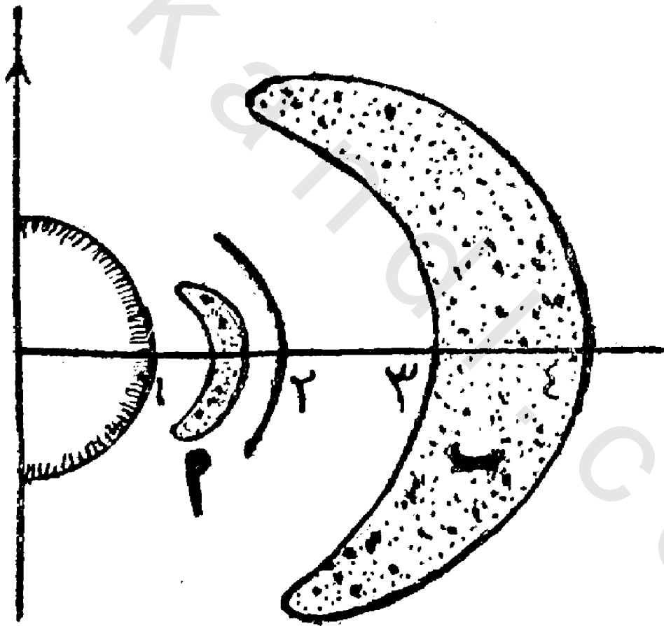
شكل ( ١٦ ) أحزمة فان آلين الإشعاعية من حول الأرض ١ — حزام فان آلين الداخلى ٢ — حزام فان آلين الخارجى
