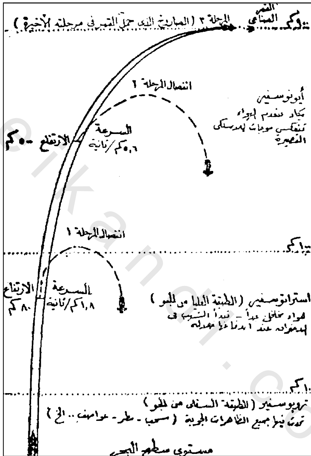
شكل (٨) صاروخ من ثلاثة مراحل استخدمه الروس في إطلاق القمر الصناعي الأول
