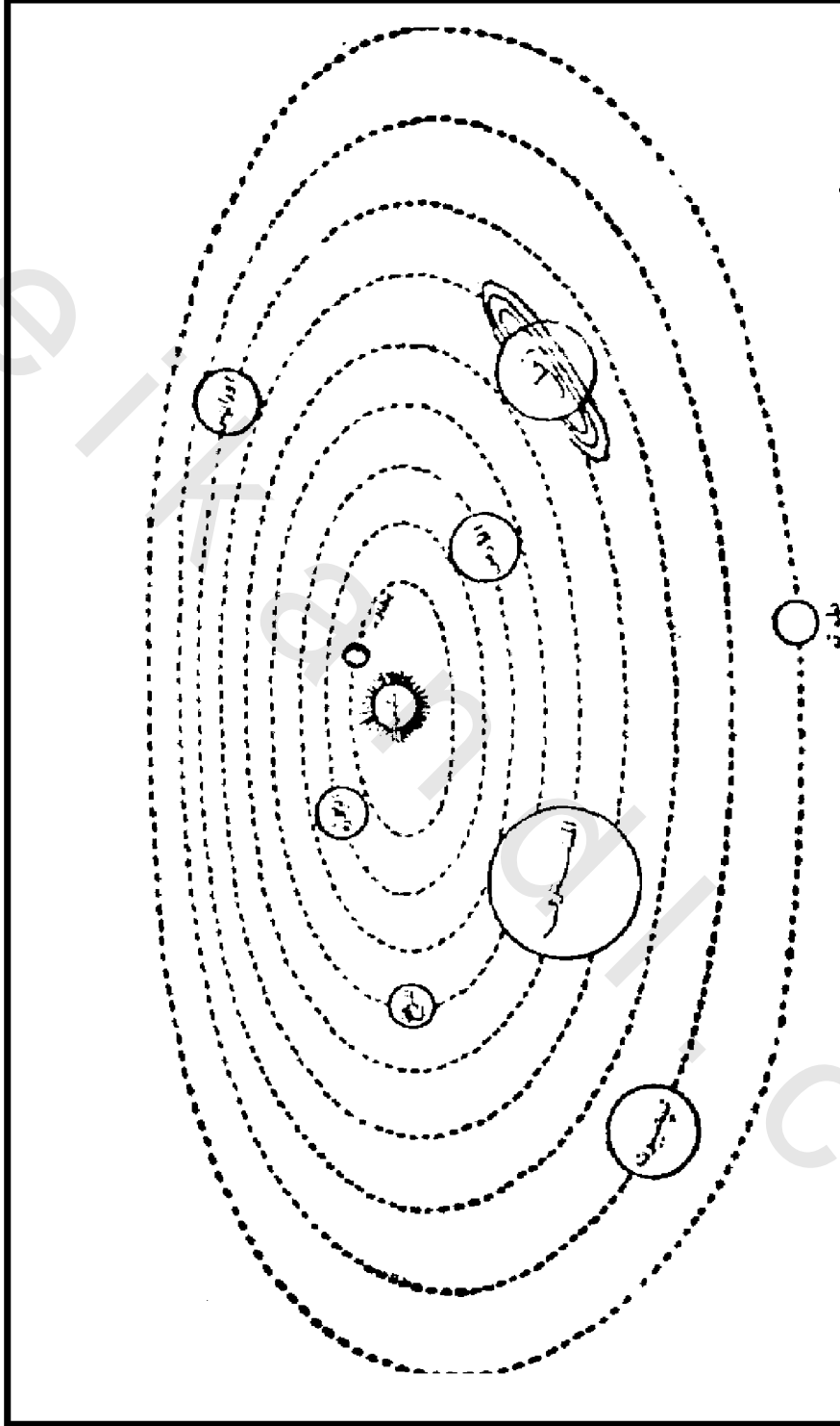
شكل ( ٢ ) أفراد المجموعة الشمسية
