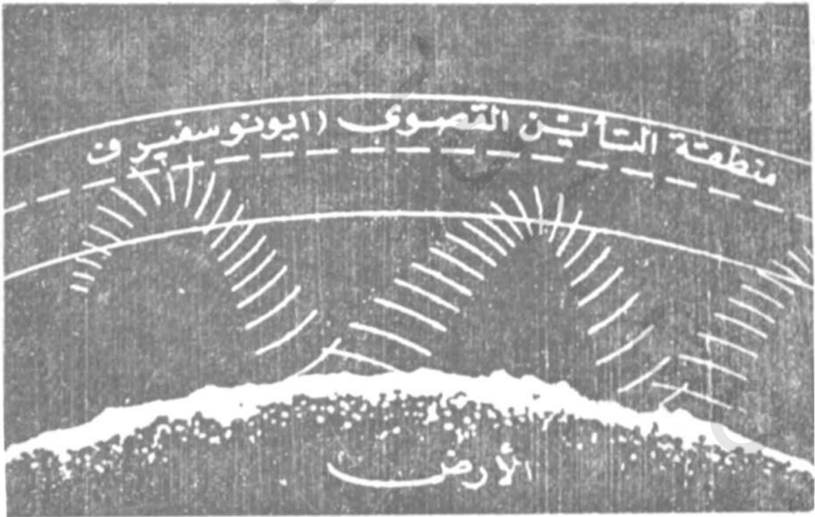
شكل (١٧) ارتداد أمواج الأثير من الطبقة ف .
