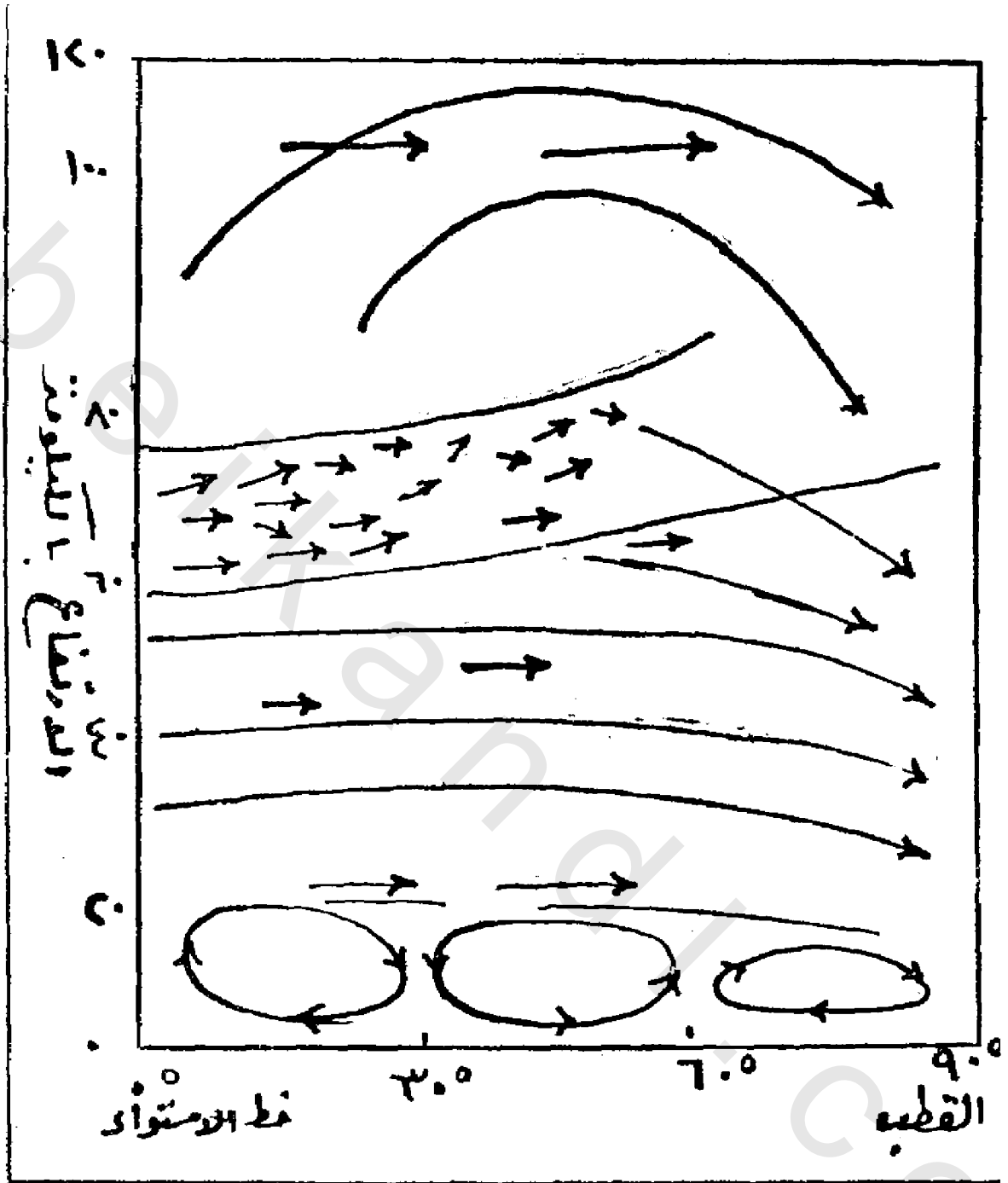
شكل (١٥) يمثل توزيع الرياح إلى علو ١٢٠ كيلو مترا فوق السطح في نصف الكرة الشمالي في الشتاء
