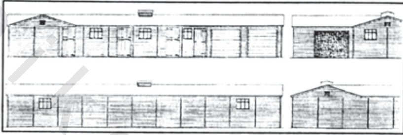
شكل (٢٥) : البوكسات ذات المبنى كامل الغلق
