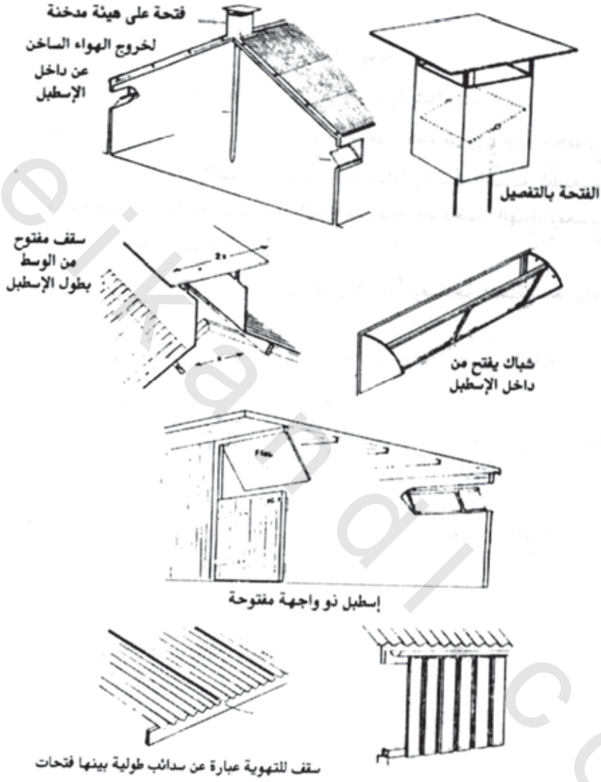
شكل (٢٧): وسائل التهوية بالمبنى
