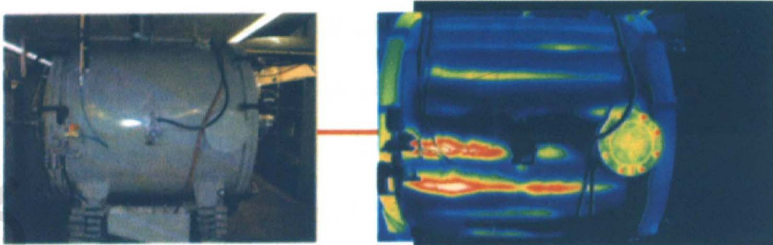
شكل رقم ( ٧ ) : تحديد الانسداد فى دوائر التبريد بالأفران.
