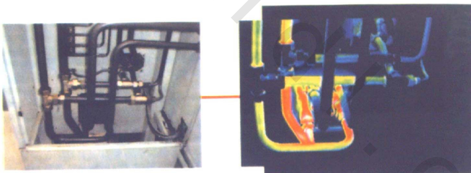
شكل رقم ( ٨ ) : تحديد أماكن الانسداد الجزئى لمواسير ضخ الزيت فى الدوائر الهيدروليكية .
