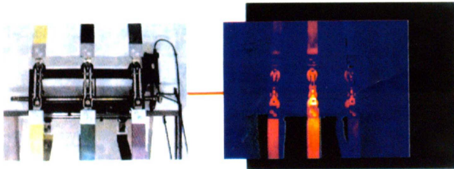
شكل رقم ( ١٠ ) : تحديد مواقع ارتفاع درجة حرارة الموصلات وقضبان التوزيع الكهربائية بسبب الأطراف غير محكمة الربط .
