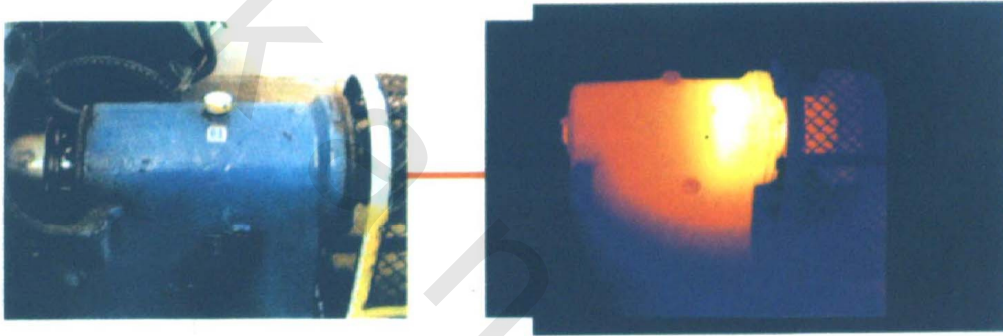
شكل رقم ( ٦ ) : التنبؤ بأعطال طلبات المياه بمعرفة مدى سخونة نقاط الارتكاز (رولمان بلى) لمحور الطلبة.
