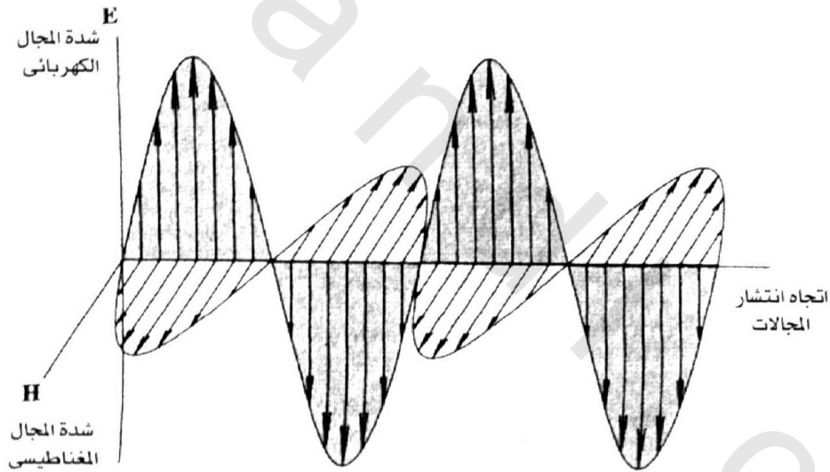
شكل رقم (١) : الموجة الكهرومغناطيسية تتكون من موجة كهربائية متعامد عليها موجة مغناطيسية وتنتشر فى اتجاه عمودى على الموجتين.
