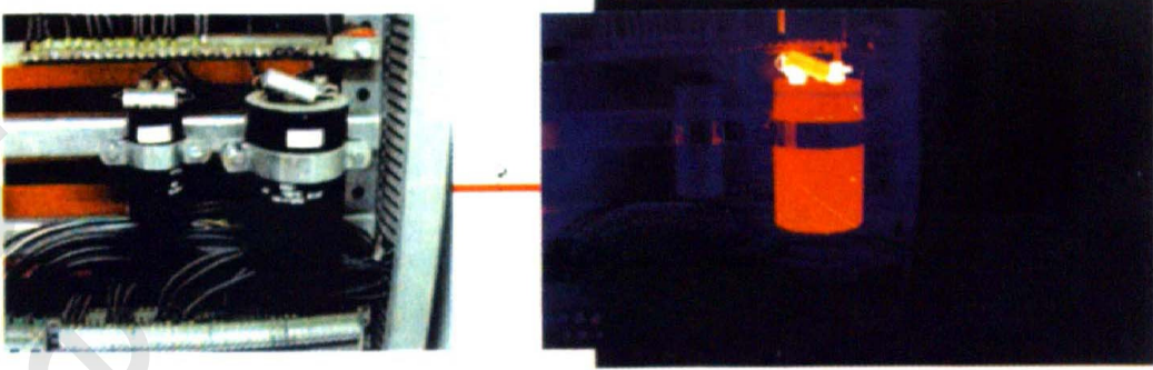
شكل رقم (١١) : صورة توضح توقع حدوث انفجار بأحد المكثفات الكهربائية.
