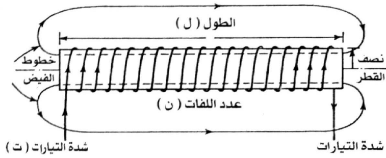
شكل ( ٧ - أ ) ملف مستقيم للحصول على مجال مغناطيسي قوى .
