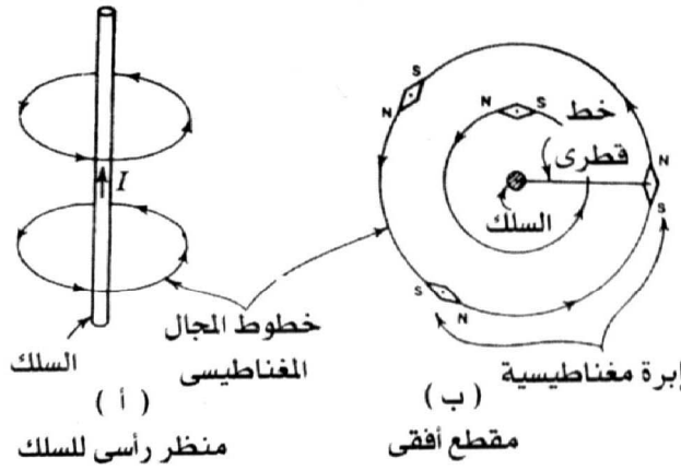
شكل رقم ( ٦ ) المجال المغناطيسى الدائرى حول سلك يحمل تياراً كهربائياً.
