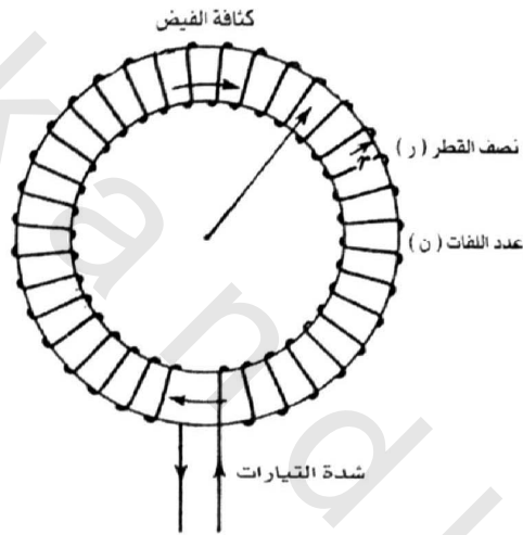
شكل ( ٧ - ب ) ملف دائري للحصول على مجال مغناطيسي قوى .
