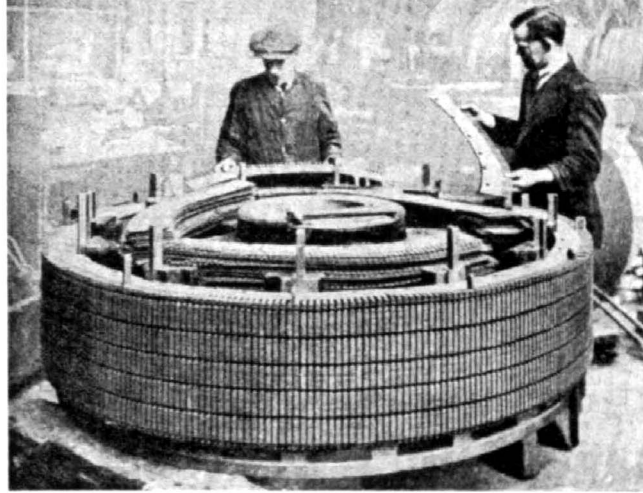
شكل (٤) الجزء الدوار لآلة كهربائية كبيرة.
