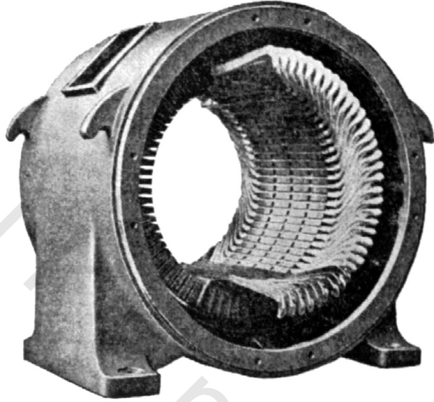
شكل (٥) ملفات مدفونة داخل مجارى محفورة.
