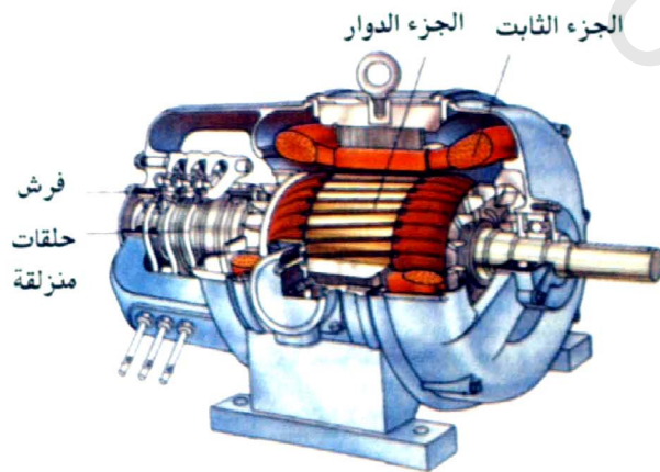
شكل (١١) محرك ذو حلقات منزلقة.
