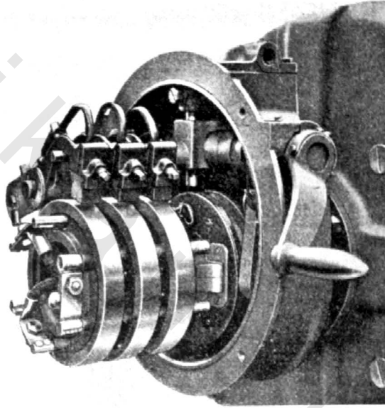
شكل (١٣) صورة توضح الحلقات المنزلقة في محرك القفص السنجابي.
