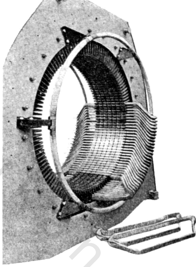
شكل (٣) يوجد داخل الجزء الثابت مجموعة ملفات كهربائية مدفونة داخل مجارى محفورة في السطح الداخلي للجزء الثابت (لاحظ عدد ٢ ملف منفرد أسفل الجزء الثابت للآلة).
