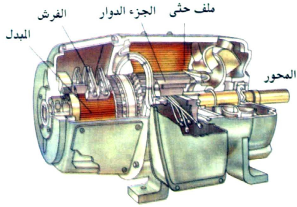
شكل (٩) محرك تيار مستمر.
