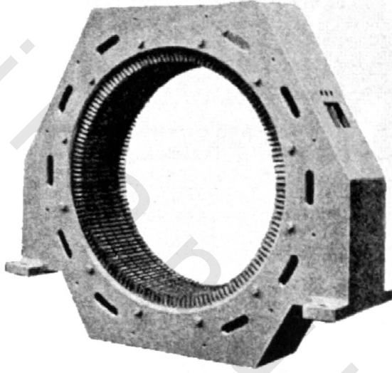
شكل (١٥) الجزء الثابت لمولد كهربائى عالى القدرة.
