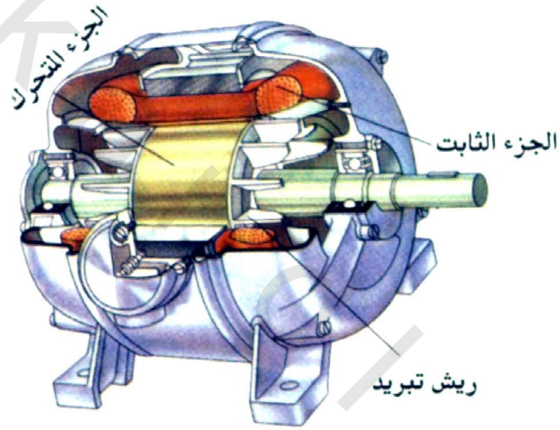
شكل (١٠) محرك ذو قضب سنجابي.
