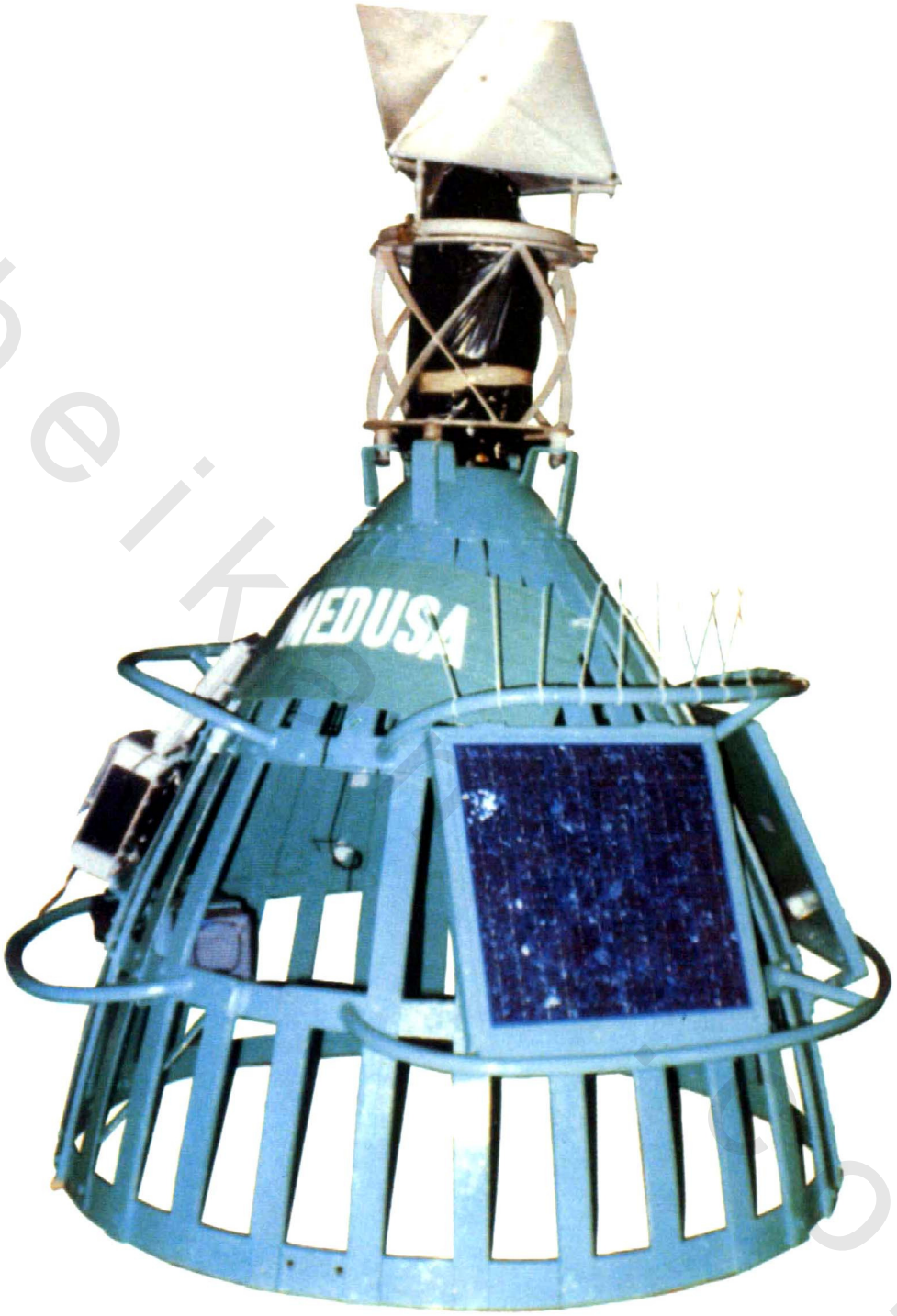
شكل ( ٢٠ ) جهاز يركب على العوامات البحرية (الشمندورة) لإثارتها ليلا حتى تقوم بإرشاد السفن - وهذا الجهاز يعمل بالطاقة الشمسية .
