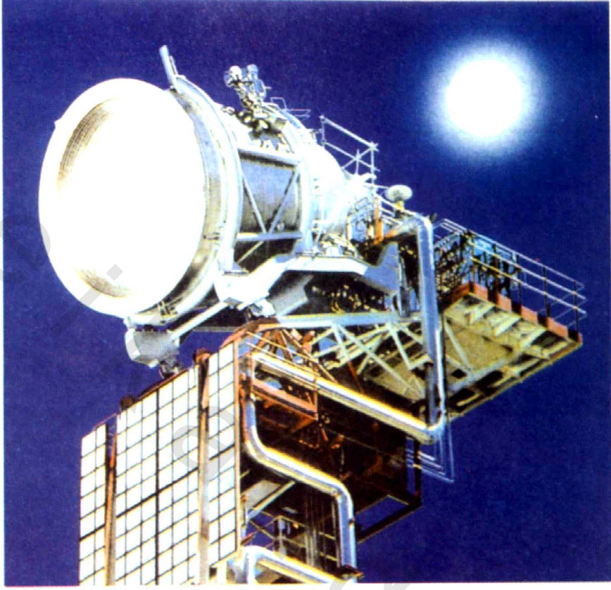
شكل ( ٩ ) بوتقة صهر المعادن أو ( أم النار )
