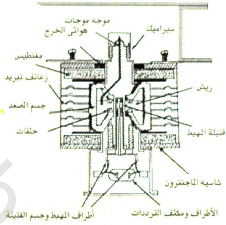
شكل رقم (٤ هـ) مقطع فى الماجنترون
