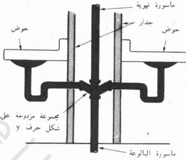
الشكل رقم ١/١٤: وحدة تهوية تستخدم جهازين متماثلين يتم تركيبها ظهراً لظهر
