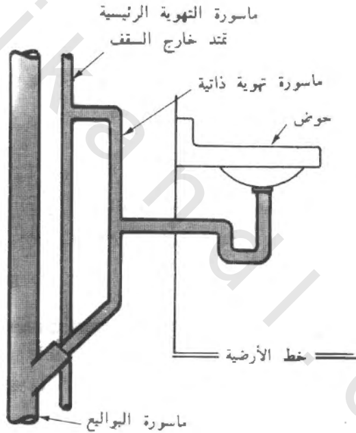
الشكل رقم ١٣/١ Masura تهوية ذاتية تمنع تقريباً احتمالات فقدان مياه محبس الروائح الذي يعمل كمانع للتسرب
