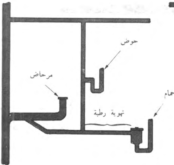
الشكل رقم ١/١٨ يمكن إقامة المهوئات الرطبة لخدمة الأجهزة التي يكون التفريغ فيها للسوائل فقط
