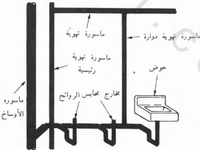
الشكل رقم ١/١٥ تقام المهيويات الدائرية على الفروع الأفقية لخدمة جهازين أو أكثر
