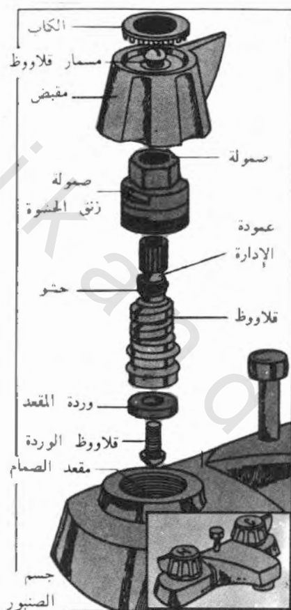
الشكل رقم ٢/٧ صنبور الضغط
