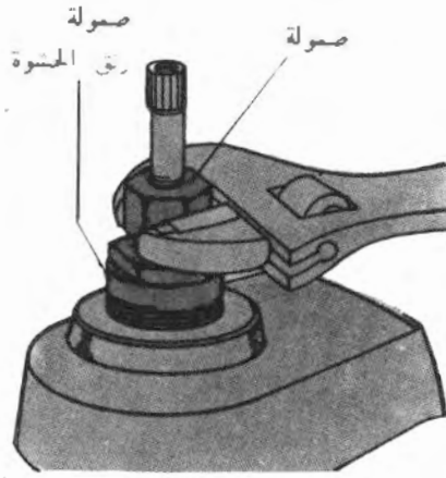
الشكل رقم ٢/٨ لفك الصنبور إلى أجزاء متفرقة استخدم مفتاحاً هلالياً في حلّ صمولة الساق وصمولة زئق الحشوة
