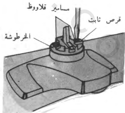
الشكل رقم ٢/١٦ راجع موانع التسرب لتغير التالف منها
