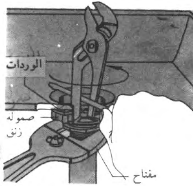
الشكل رقم ٣/١٠ لربط صمو له الزئق للمصفاة: - استخدم زردية ومفكاً
