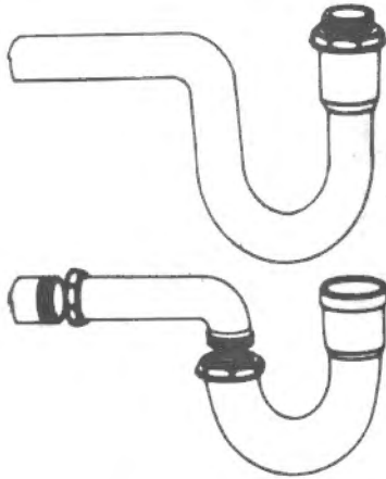
الشكل رقم ٣/٢٢ - أنواع مختلفة من محابس الروائح
