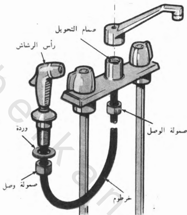
الشكل رقم ٣/١ رشاش الحوض، صمام التحويل
