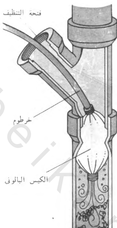
الشكل رقم ٣/٣٧ استخدام الكيس البالوني لتسليك المواسير
