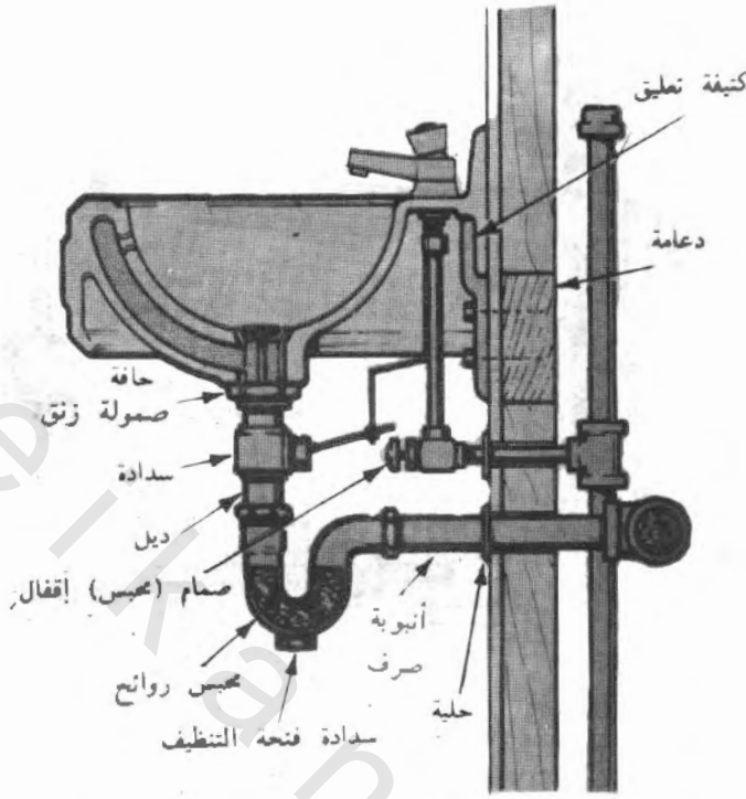
الشكل رقم ٣/١١ نموذج غطى لحوض محمول على الحائط موضحاً فيه سدادة Pop-up وصمامات الإقفال
