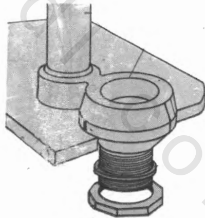
الشكل رقم ٤/١٦ لتركيب أنبوبة تصريف الفائض أعد تثبيت صمولة الزنق
