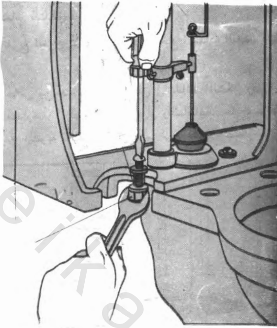
الشكل رقم ٤/١٥ خزانات فوق السلطانية: يوجد لها عدد ٢ مسمار قلاووظ تقوم بتوصيل الحزان فوق اللطانية
