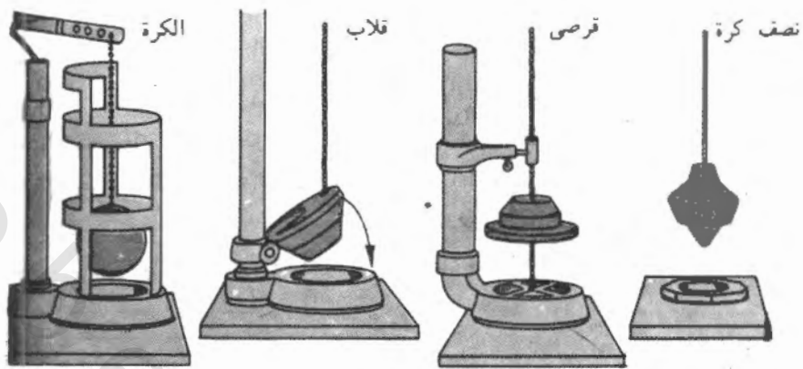
الشكل رقم ٤/١٢ سدادات الخززان: الكرة، قلاب، قرصى، نصف كرة
