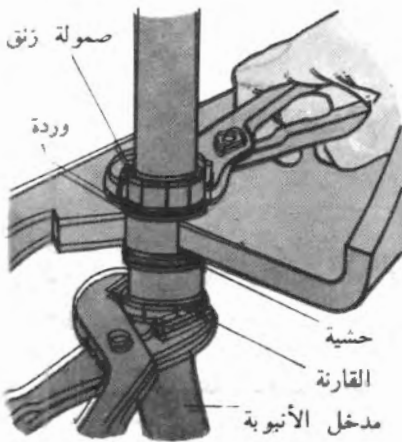
الشكل رقم ٤/٨ لحلّ مجموعة المحبس الكروي استخدم مفتاحين
