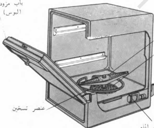
الشكل رقم ٥/١٤ جهاز غسالة الصحون
