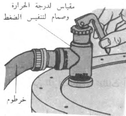
الشكل رقم ٥/١٢ لاختبار مقياس درجة الحرارة وصمام تنفيس الضغط ارفع مقبض الصمام حتى يتم تصريف الماء الساخن
