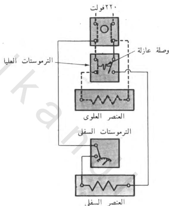
الشكل رقم ١٠/٥ نظام توزيع الأسلاك فى سخان المياه الكهربى
