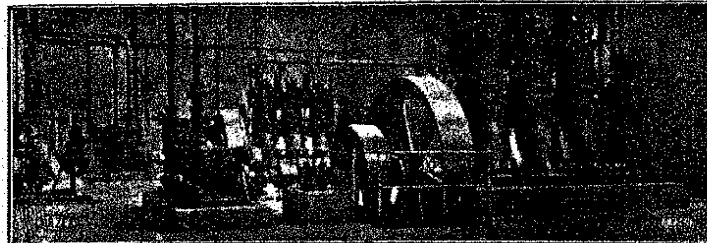
بمعمل ثلج بيورسميد يشتغل بمكبس للشادر طرز سولزر ( ٦٠٠٠ و ٦٠٠٠٠ ) بمبرد انكليزي بالساعة ) يدار بواسطة محركات طرز سولزر ديزل قوتها الاجالية ٢٤٠ حصانا
