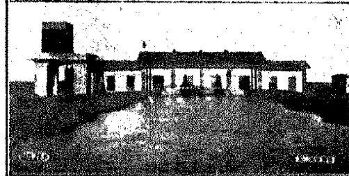
مخمة طلمبات البصري للصرف مشتملة على اربع طلمبات عمود طرز سولزر ديزل بقوة ١١٠٠ حصاناً
