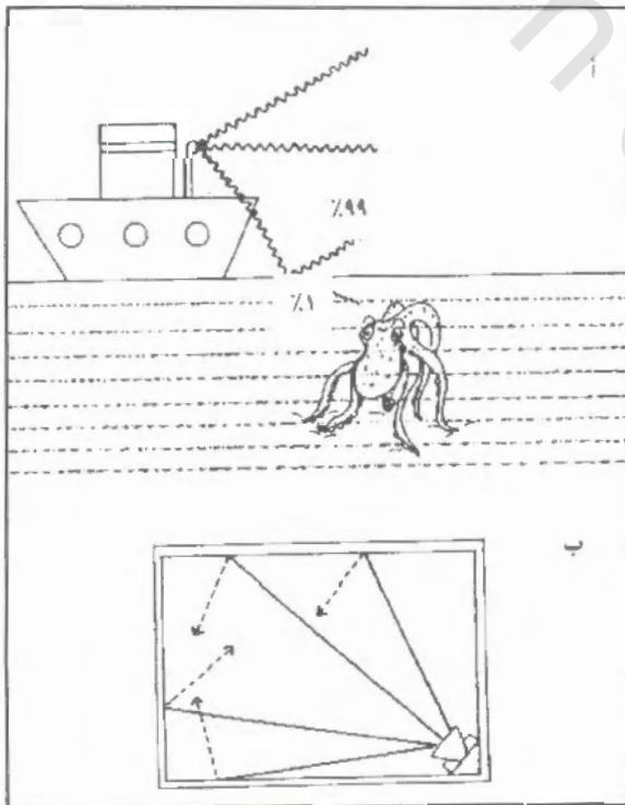
(شكل ١٣) عند اصطدام موجات الصوت بالسطح الفاصل بين وسطين مختلفين، فإن غالبيتها ينعكس ولا يمر خلال الوسط الثانى إلا قدر ضئيل جداً منها.
