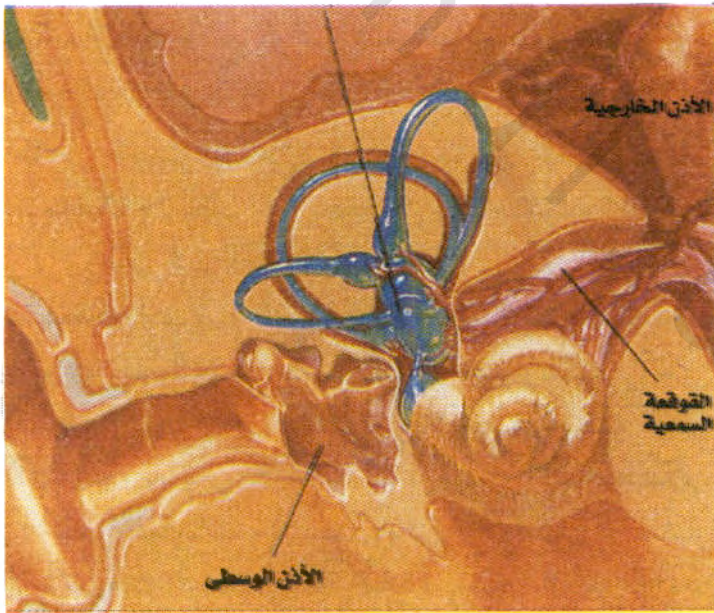
(شكل ٩) تركيب الأذن البشرية : الأذن الخارجية ثم الوسطى فالداخلية (القوقعة السمعية).
