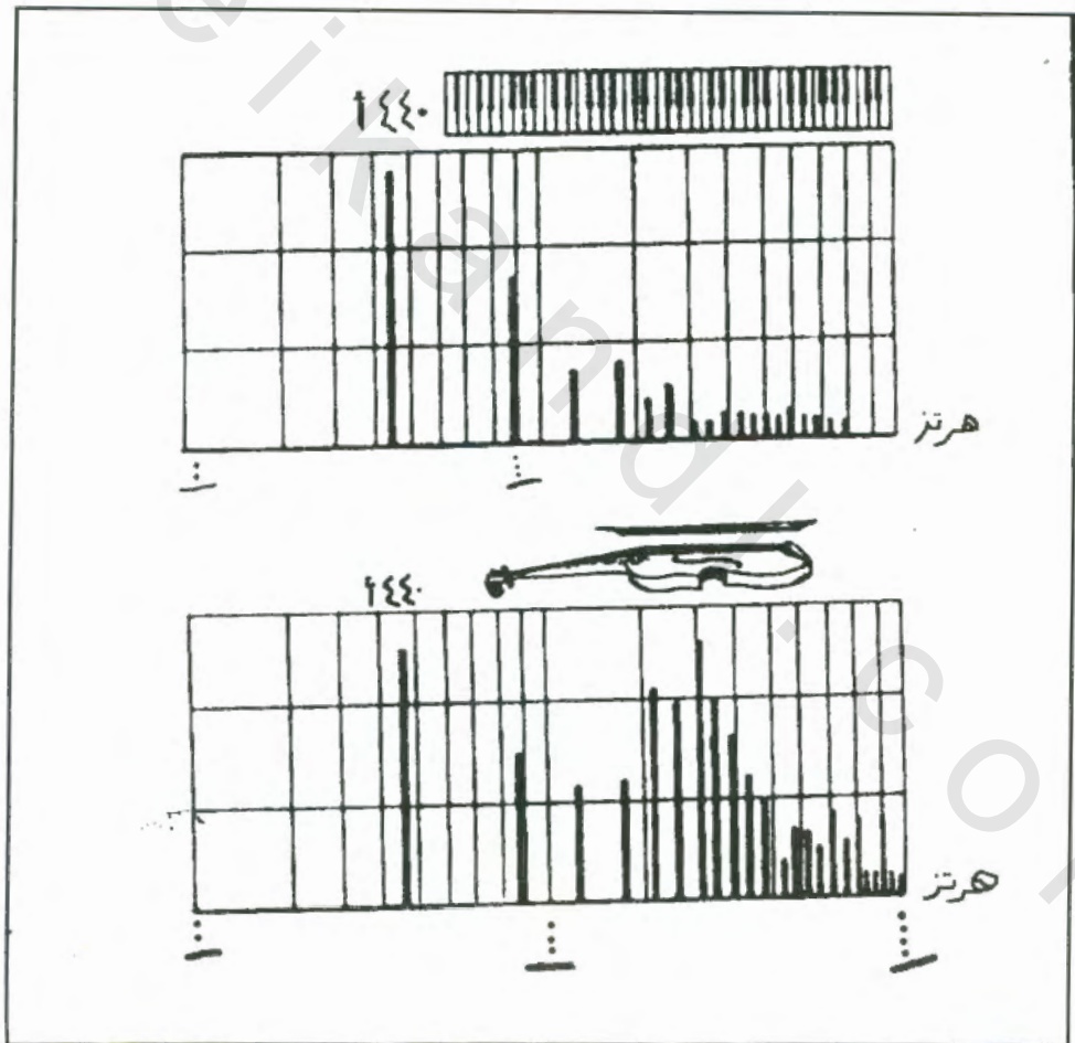
( شكل ٨ ) رسم توضيحي لكيفية تحليل النغمات المعقدة المختلطة الصادرة عن آلة صوتية (الكمان والبيانو هنا)، إلى وحداتها الأساسية من نغمات صوتية بسيطة ذات ترددات مختلفة ( تحليل الصوت ).
