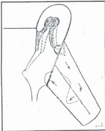
(شكل ١٢) هكذا تهز موجات الصوت غشاء الطبلة وعظيومات الأذن الوسطى، مما يسبب تحرك السوائل المضغوطة فى الأذن الداخلية، مما يذبذب الخلايا العصبية لعضو كورتى، وتتحول الذبذبات إلى نبضات كهربية ينقلها عصب السمع للمخ.
