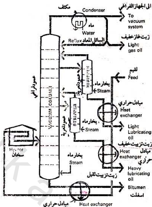
وحدة تقطير فراغي
