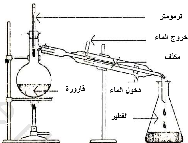
جهاز معملّي للتقطير البسيط
