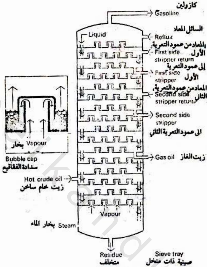
مقطعاً من عمود التجزئة وتركيب الصواني
