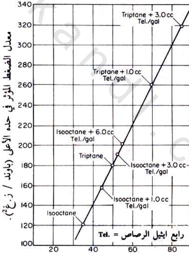
العلاقة بين القدرة الناتجة وضغط زيادة الشحنة
