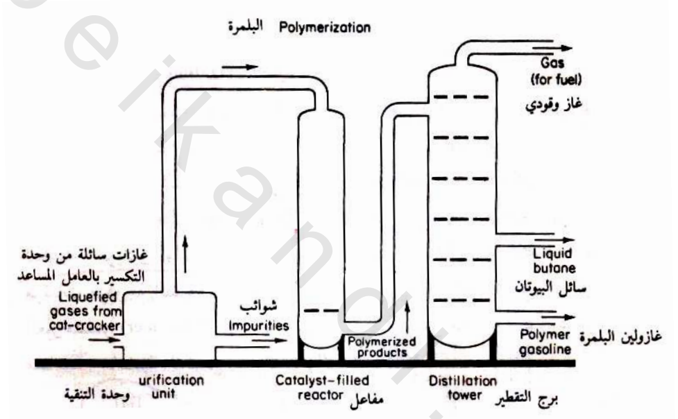
مخطط وحدة البلمرة الصناعية
