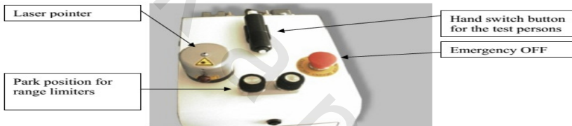
شكل رقم (٣٩) يوضح ضبط مكونات الديناموميتر من أعلى
