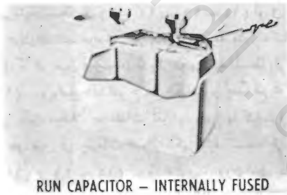
رسم رقم (٢ - ٢٠) - كباستور الدوران ويظهر المصهر المركب داخل علبة
