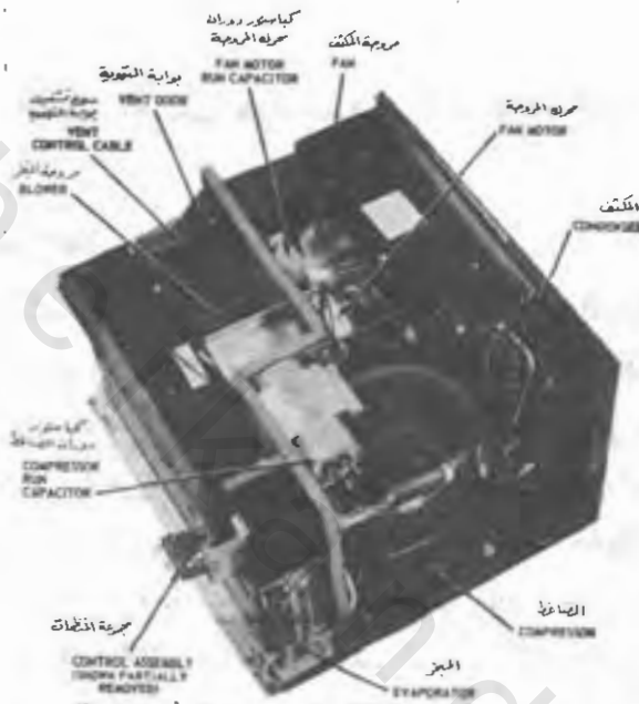
رسم رقم (٢ - ١) - الأجزاء الأساسية التي يتركب منها جهاز تكييف هواء الغرف
