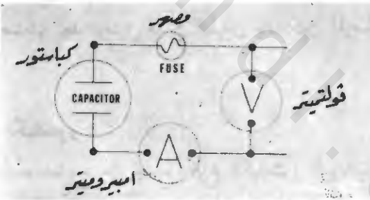
رسم رقم (٢ - ٤٠ أ) - طريقة توصيل جهاز الفولتيتر وجهاز الأمبيروميتر في دائرة اختبار سعة الكباستور .
