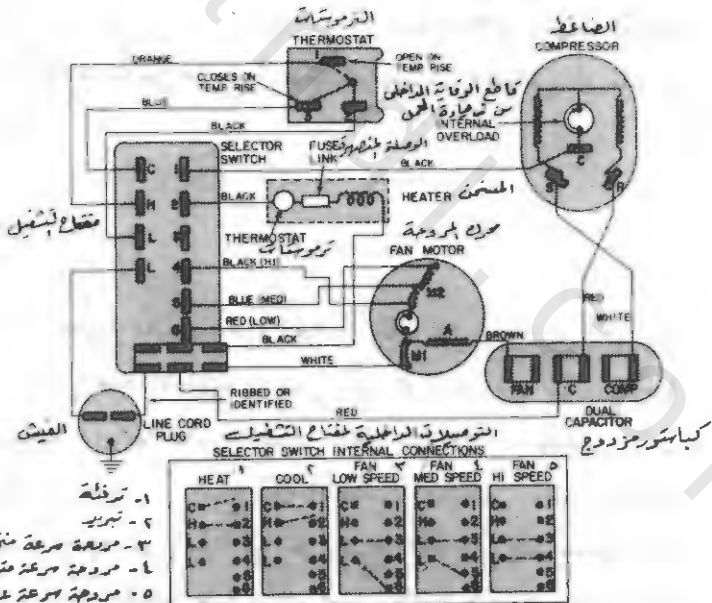
رسم رقم (٢ - ١٢٥) - الدائرة الكهربائية البسيطة لجهاز تكييف هواء، غرف مركب به مسخن كهربائي للتدفئة وطريقة توصيله بالدائرة.
