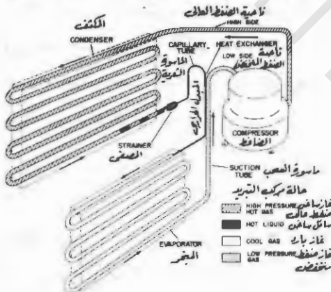
رسم رقم (٢ - ١) - الأجزاء الأساسية التي يتركب منها جهاز تكييف هواء الغرف
