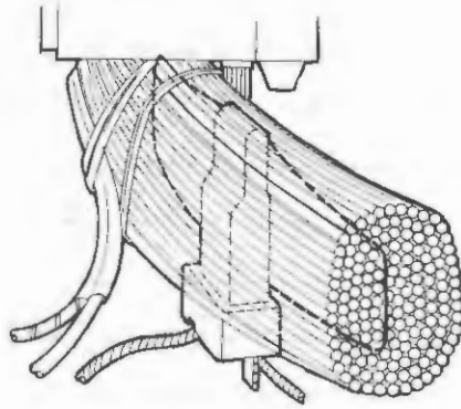
رسم رقم (٢ - ١٧) - قاطع الوقاية من زيادة حمل محرك الضاغط . من النوع الذي يركب داخل ملفات المحرك نفسه .
