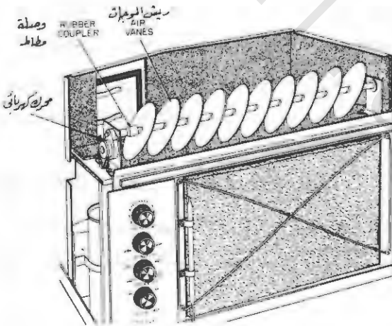
رسم رقم (٢ - ٦) - موجّهات الهواء المتحركة بجهاز تكييف هواء الغرف
