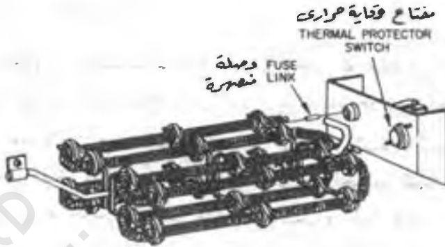
رسم رقم (٢ - ٢٥) مسخنات تدفئة الهواء ومركب معها مفتاح الوقاية الحرارية والوصلة المنصهرة
