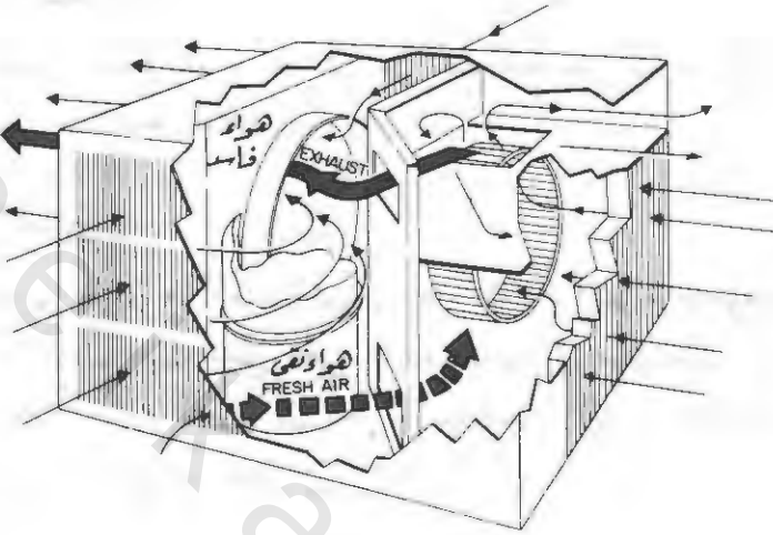
رسم رقم (٢ - ٥) - اتجاه حركة الهواء بجهاز تكييف هواء الغرف
