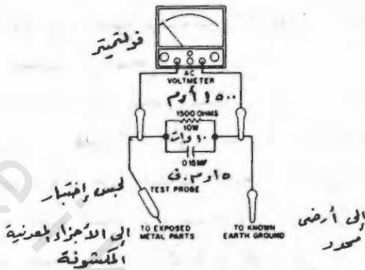
رسم رقم (٢-٢٦) - دائرة اختبار تسرب التيار
