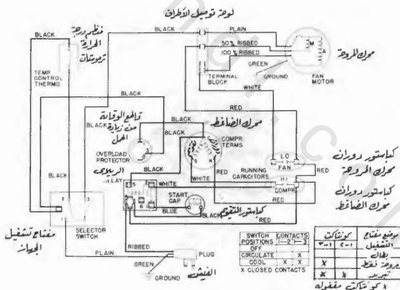
رسم رقم ( ٢ - ١٤ ) - الدائرة الكهربائية المبطة لجهاز تكييف هواء الغرف يشتمل على ريلاي تقويم لحركه الضاغط من النوع الذى يعمل بتأثير الفولت
