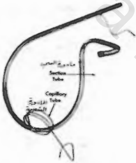
رسم رقم ( ٢ - ٥٨ ) الأجزاء التي يتركب منها المبدل الحرارى
