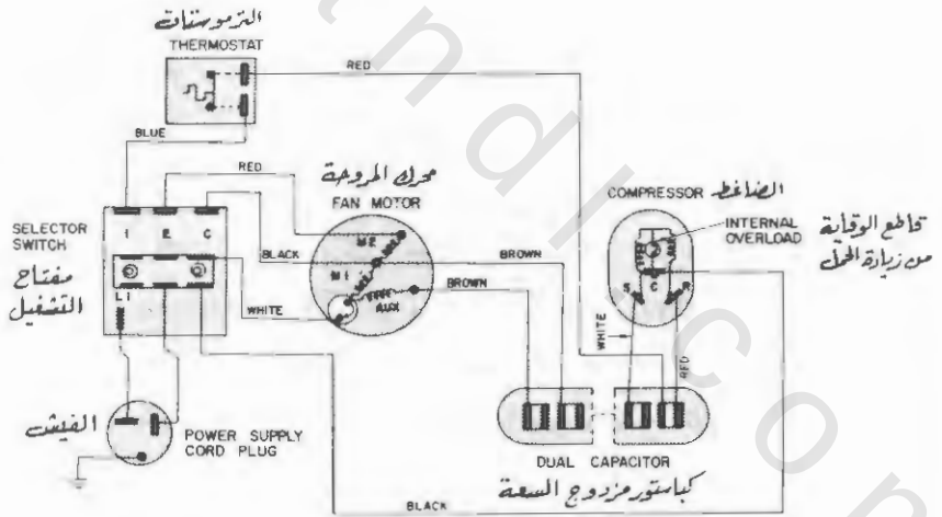
رسم رقم (٢ - ١٨) - الدائرة الكهربائية المبسطة لمحرك تكييف هواء غرف من النوع الذي يشتمل على محرك ضاغط مركب داخل ملفاته قاطع وقاية من زيادة الحمل .
