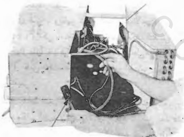
رسم رقم ( ٢ - ٤٥ ) - طريقة اكتشاف التنفيس باستعمال لمبة التجربة من نوع الهاليد .
