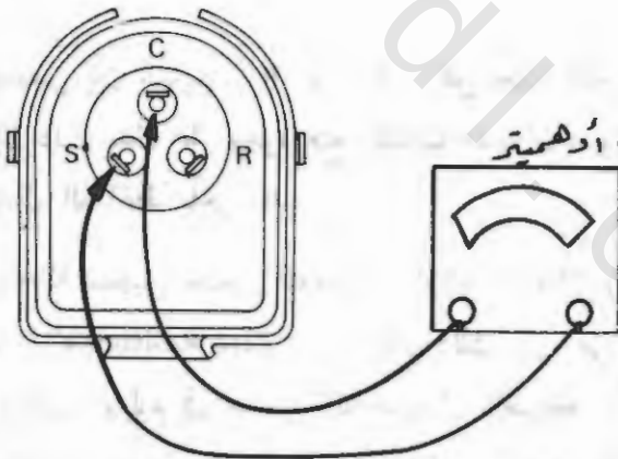
رسم رقم ( ٢ - ٣٢ ) - التأكد من أن ملفات محرك الضاغط سليمة باستعمال جهاز أوهميتر
