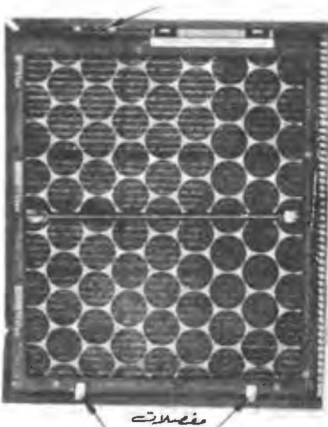
رسم رقم ( ٢ - ٩ ) مرشحات الهواء التي يلزم تغييرها من وقت لآخر والمصنوعة من نسيج الشعر الزجاجي . وتبين هذه الصورة طريقة تركيبها في البرواز الخاص بها .
