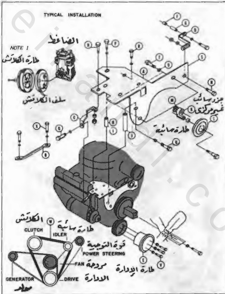
رسم رقم ( ٧١-٩ ) - أماكن تركيب الجزء السائب الغير مركزى ، والطارة السائبة ، وسيور الإدارة
