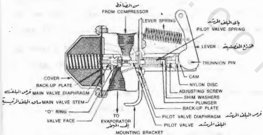
رسم رقم (٩-٣١) — قطاع في ملف تبريد الغاز الساخن يبين الأجزاء المختلفة التي يشتمل عليها
