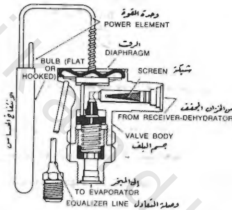
رسم رقم (٩ - ١٠) - قطاع فى بلف التمدد الحرارى ذى وصلة التعادل
