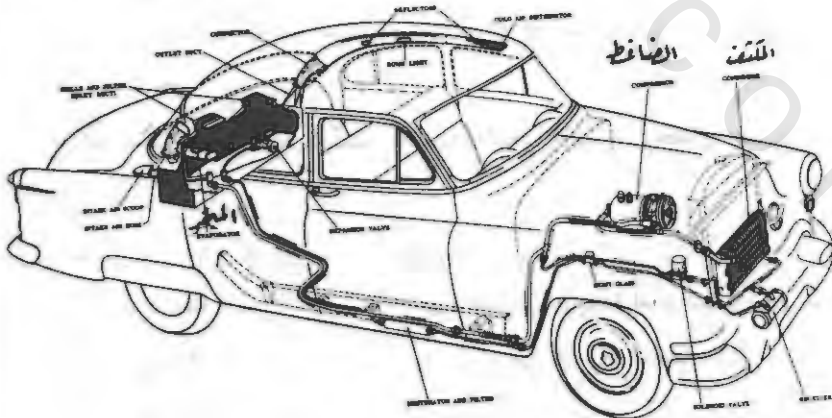
رسم رقم ( ٩ - ٥ ) - تركيب مجموعة المبخر في الحيز الخلفي بالسيارة المخصص لوضع الحقائب
