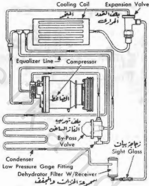
رسم رقم (٩-٣٠) — مكان تركيب ملف تبريد الغاز الساخن في دائرة تبريد جهاز تكييف هواء السيارات
