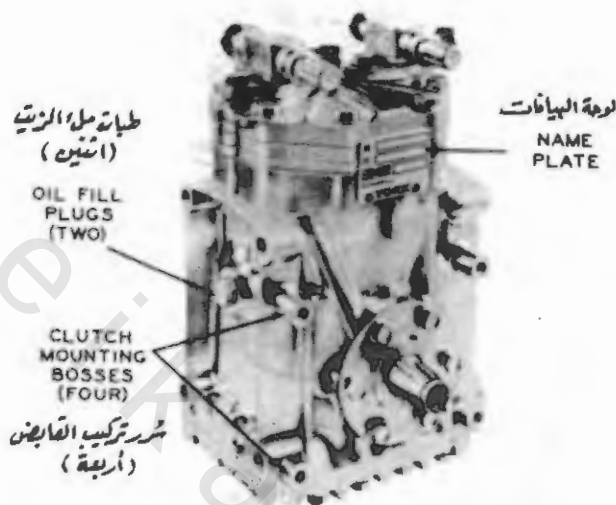
رسم رقم (٩-١٢) - الشكل الخارجى للضاغط صناعة «يورك»
