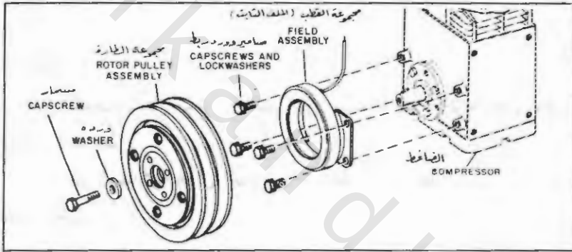
رسم رقم ( ٩ - ٢٥ ) - الشكل الخارجي للقابض الكهربائي ( الكلاش الكهربائي ) والأجزاء التي يتركب منها ، وطريقة تركيبه مع الضاغط
