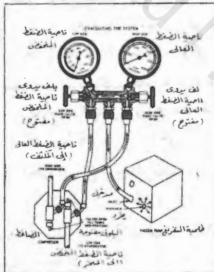
رسم رقم ( ٩ - ٤٢ أ ) - طريقة توصيل الطلبة للتفريغ بدائرة التجريد لعمل تفريغ بها
