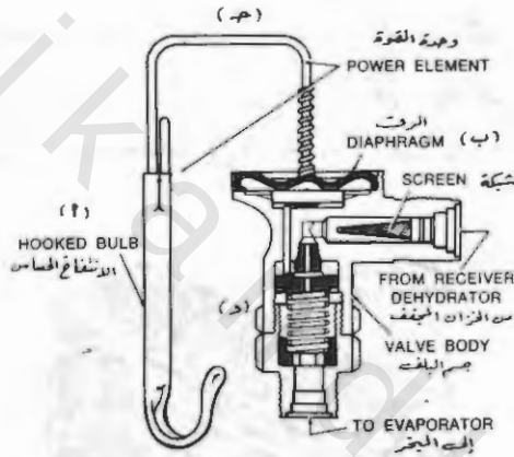
رسم رقم (٩-٩) - قطاع في بلف التمدد الحرارى تظهر به الأجزاء التى يتركب منها
