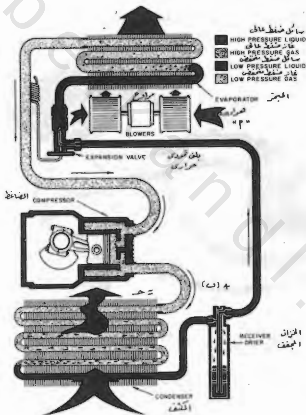
رسم رقم (٩ - ٢) كيف يعمل جهاز تكييف هواء السيارة
