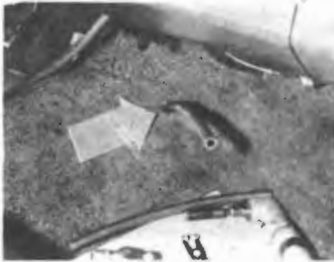
رسم رقم ( ٩ - ٧٥ ) إمرار خرطوم تصريف ماء التكاثف بأرضية السيارة
