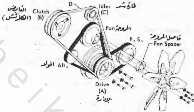
رسم رقم (٩-١١) - ترقية السيور الخاصة بإدارة الضاغط عن طريق القابض
