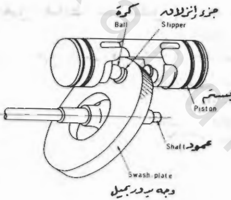
رسم رقم (٩ - ١٩) تركيب البستم والوجه الذى يدور بميل
