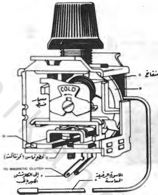
رسم رقم (٩-٣٦) - الأجزاء الأساسية التي يتركب منها ترموستات ضبط درجات الحرارة
