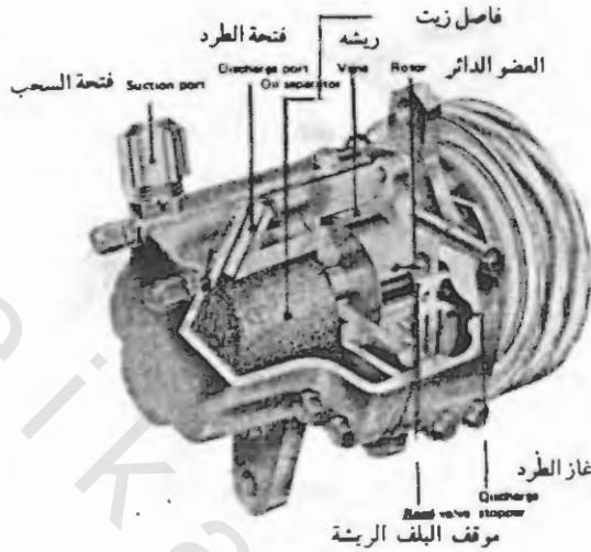
رسم رقم (٩ - ٦٠) - قطاع في الضاغط من طراز سنتروتا CPR 100.
