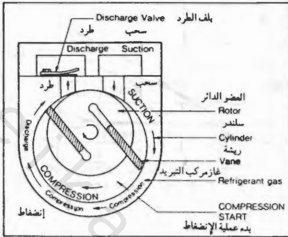
رسم رقم (٩ - ٥٧) - طريقة عمل الضاغط الدائري من طراز ماتسوشيتا الحديث.
