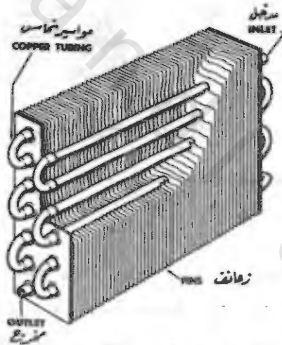
رسم رقم ( ٩ - ٨ ) - مكثف جهاز تكييف هواء السيارة من النوع الذي يشتمل على صفتين من المواشير
