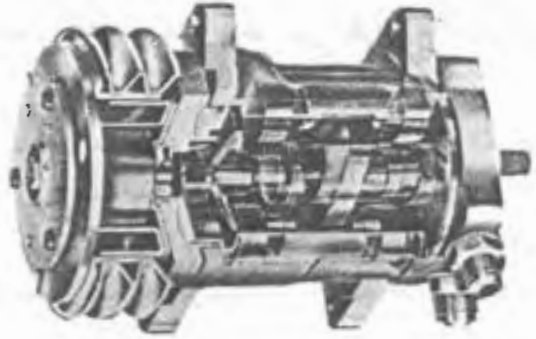
رسم رقم (٩ - ٥٤) - قطاع في ضاغط من طراز كلاريون.
