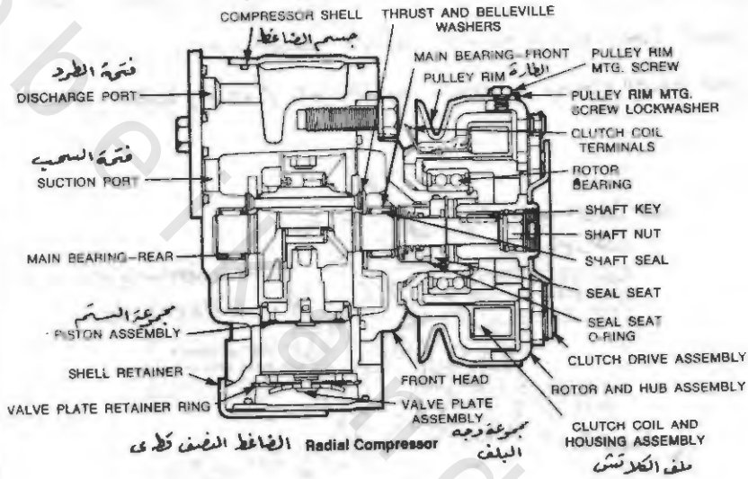
رسم رقم (٩ - ٢١) - قطاع في الضاغط النصف قطري ، تظهر به الأجزاء التي يتركب منها
