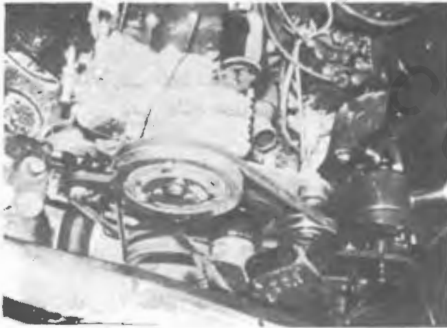
رسم رقم (٧٢-٩) - تركيب سير الإدارة حول طارة الكلاتش ، وطارة عمود المرفق ، والطارة السائبة الوسيطة
