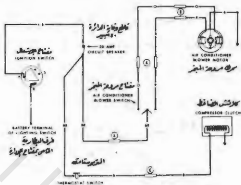
رسم رقم ( ٩ - ٢٨ ) - الدائرة الكهربائية المبسطة لجهاز تكييف هواء السيارة
