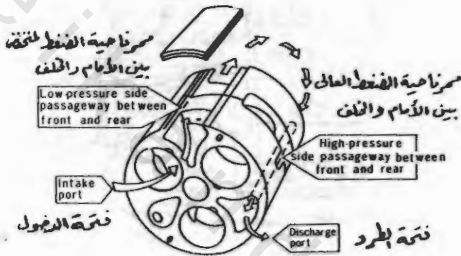
رسم رقم (٩ - ٢٠) - ممر غاز مركب التبريد
