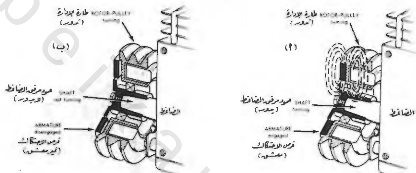
رسم رقم " (٩-٢٦) - كيف يعمل القابض الكهربائي (الكلاش الكهربائي) . (أ) عندما يكون التيار واصلًا إليه . (ب) عندما يقطع وصول التيار .
