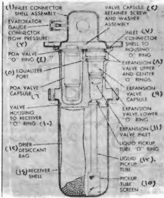
رسم رقم (٩ - ١٣٤) - قطاع في البلف في مجموعة خزان السائل (VIR)
