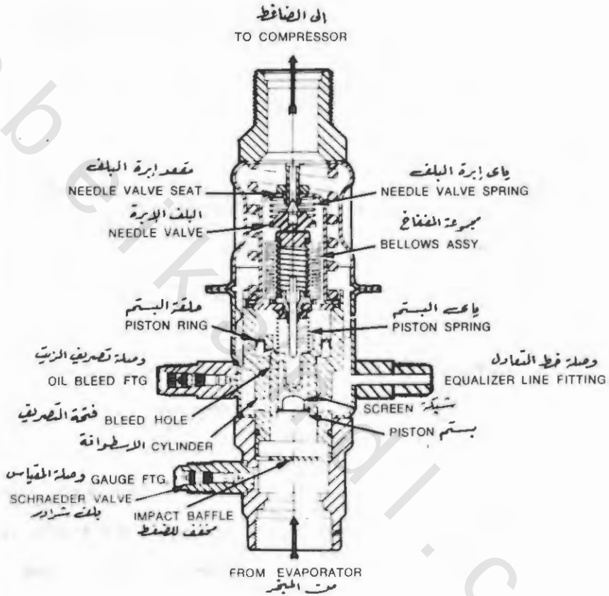
رسم رقم (٢٨-٩) - قطاع في بلف السحب الخائق المرشد المطلق بين الأجزاء المختلفة التي يشتمل عليها
