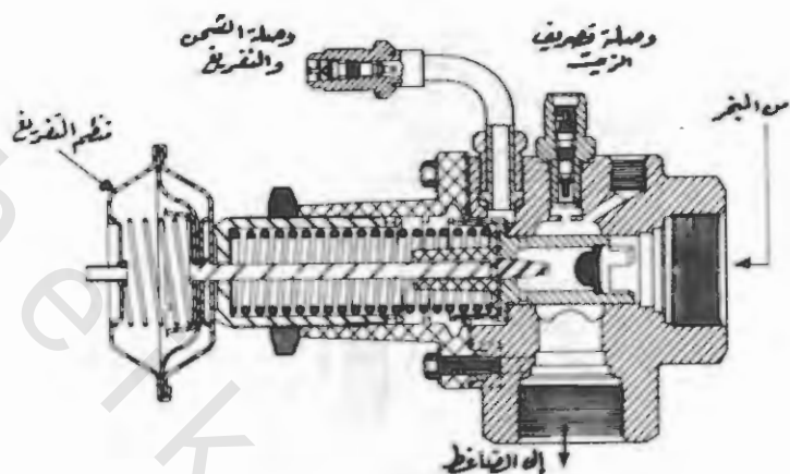
رسم رقم (٢٩-١) - قطاع في بلف السحب الخائق الذي ينظم بالتفريغ بين الأجزاء المختلفة التي يشتمل عليها
