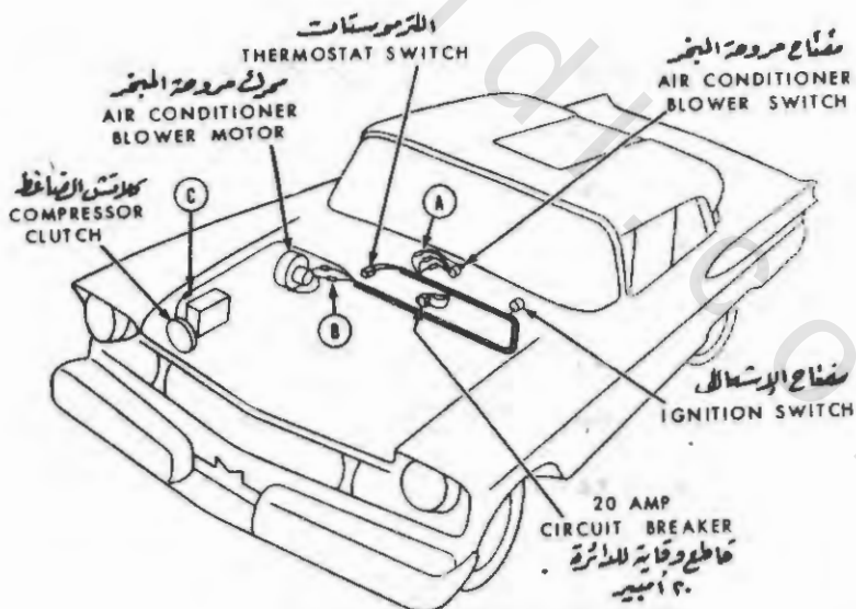
رسم رقم ( ٩ - ٣٩ ) - دائرة التوصيلات الكهربائية الخاصة بجهاز تكييف هواء السيارة
