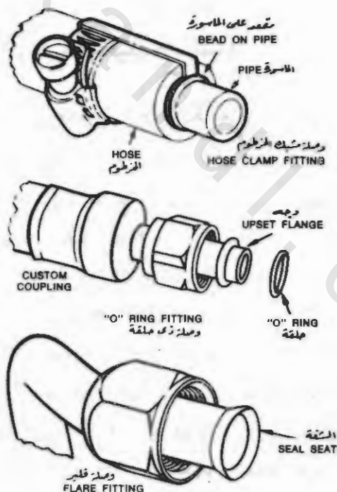
رسم رقم (٩-٣٧) - الأشكال المختلفة للوصلات التي تستعمل بخطوط دوائر التبريد الخاصة بأجهزة تكييف هواء السيارات
