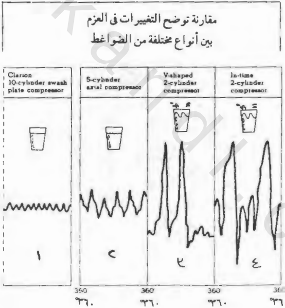
رسم رقم (٩ - ٥٥) - مقارنة توضع التغيرات في العزم بين أنواع مختلفة من الضواغط.
