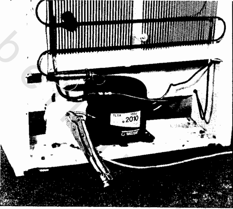
رسم رقم (١٣-٤٧) - عمل نفث بماسورة التفريغ والشحن بواسطة الزرادية الخاصة التي تظهر بالرسم
