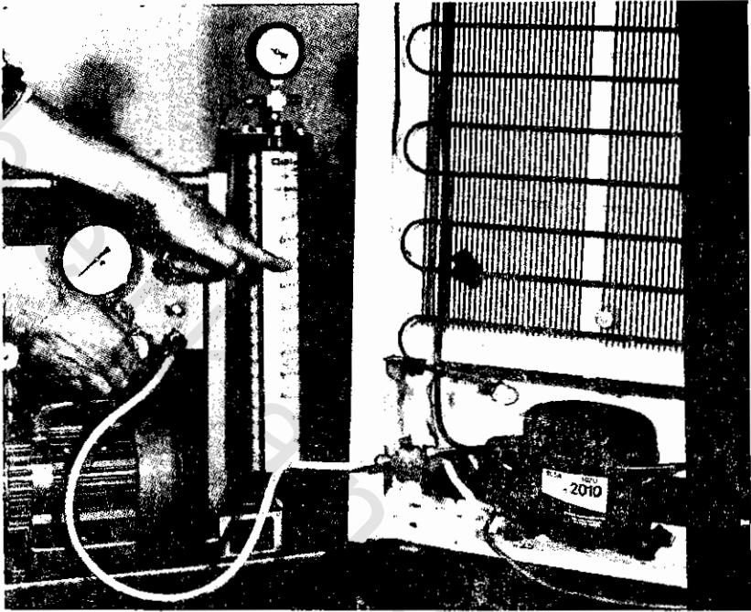
رسم رقم (١٣-٤٦) - شحن دائرة التبريد بمركب التبريد.
