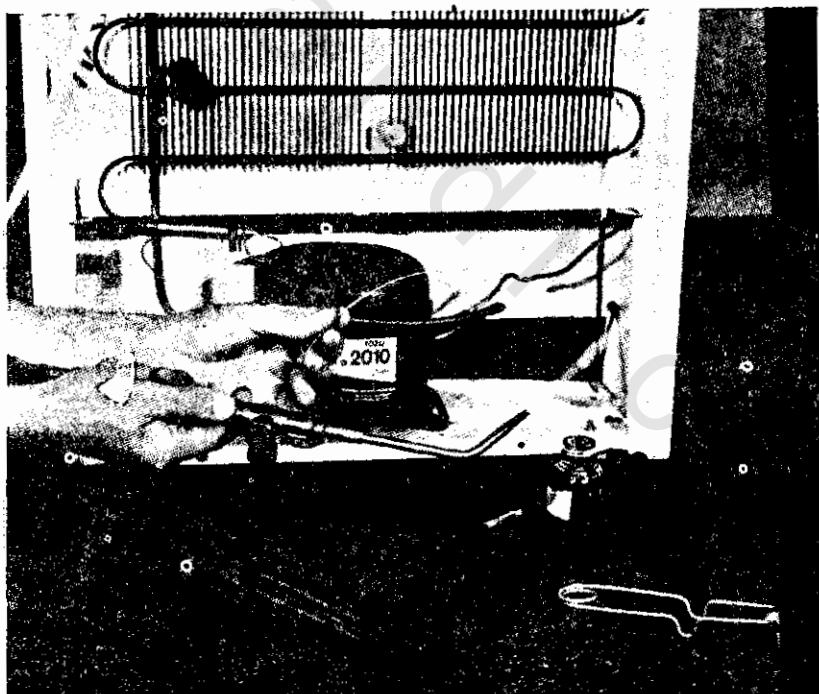
رسم رقم (١٣-٣٩) - لحام وصلات المواسير
