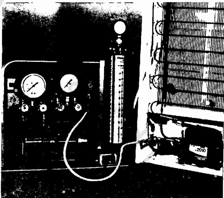
رسم رقم (١٣ - ٤٠) - توصيل طلمبة التفريغ بماسورة التفريغ والشحن الموجودة بالفضاغط
