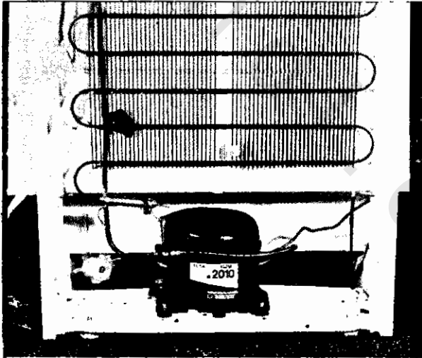
رسم رقم (١٣-٣٨) - المجفف الذى يركب بدائرة التبريد بعد فتحها
