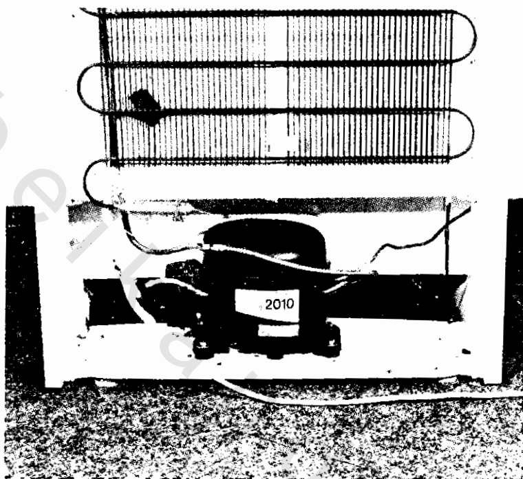
رسم رقم (١٣ - ٤٩) - تكون الآن عملية استبدال الضاغط التالف بأخر جديد قد تمت
