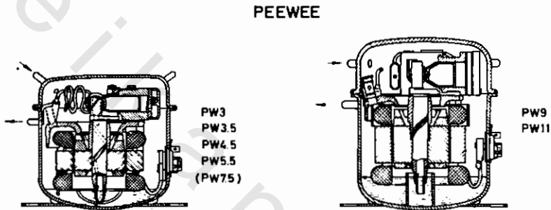
رسم رقم (١٣-١) - قطاعات فى الأنواع المختلفة من الضواغط طراز PW
