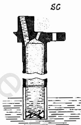
رسم رقم (١٢-١٣) - طلمبة الزيت الخاصة بالضواغط من طراز SC ، ويلاحظ وجود ريش دافعة مركبة بنهاية ماسورة سحب الزيت
