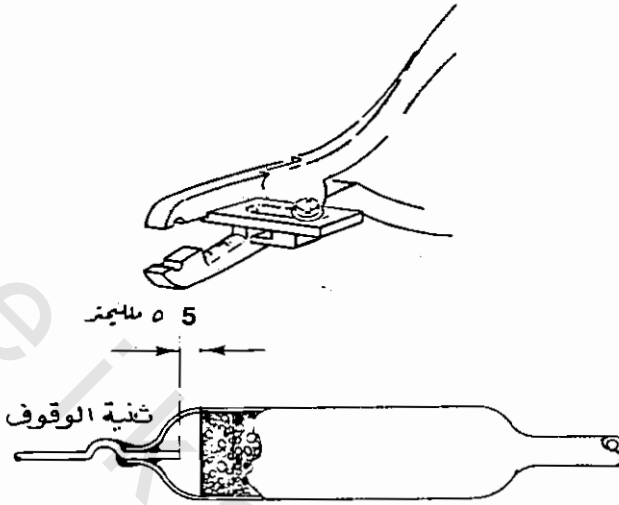
رسم رقم (١٣-٣٧) - إدخال الماسورة الشعرية داخل المرشح . وتظهر بأعلى الرسم الزرادية الخاصة بعمل شنية الوقوف
