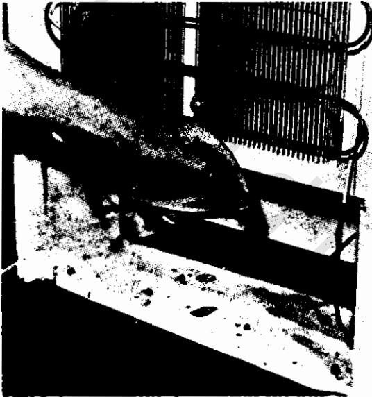
رسم رقم (١٣-٣٥) - إمرار غاز نيتروجين جاف خلال دائرة التبريد
