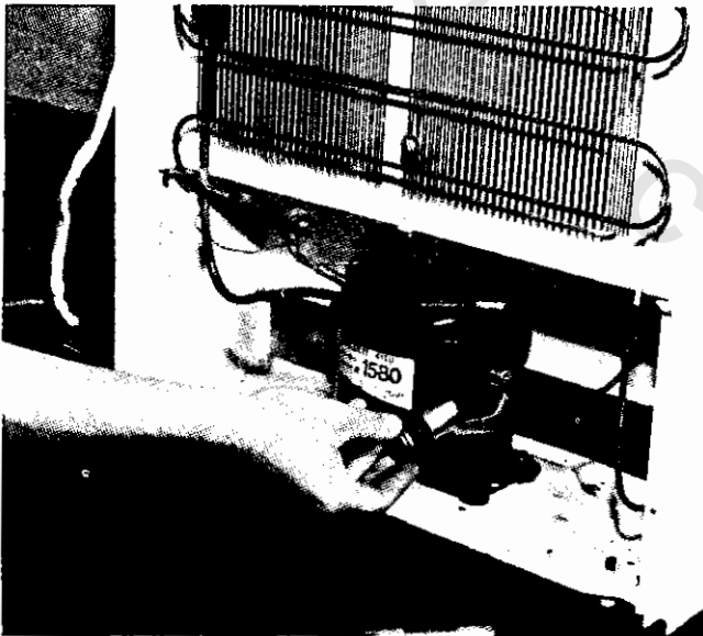
رسم رقم (٣٢-١٣) - فك الضاغط التالف باستعمال قطعة المواسير
