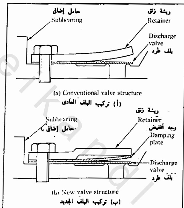
رسم رقم (١٣ - ٥٥) - مقارنة بين تركيب البلف العادى، والبلف الجديد
