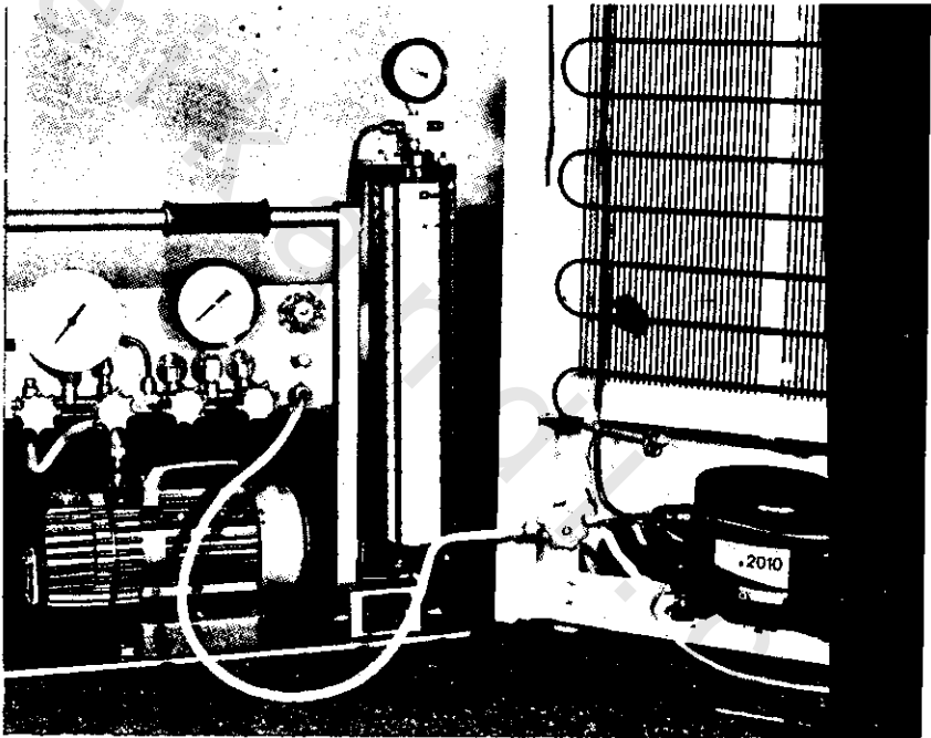
رسم رقم (٤٤-١٣) - تركيب وتوصيل
