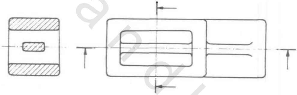
شكل "٧-٨" عدم تهشيراً أعصاب التقوية
