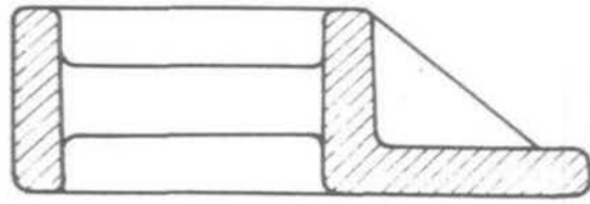
شكل "٧-٨" عدم تهشيراً أعصاب التقوية
