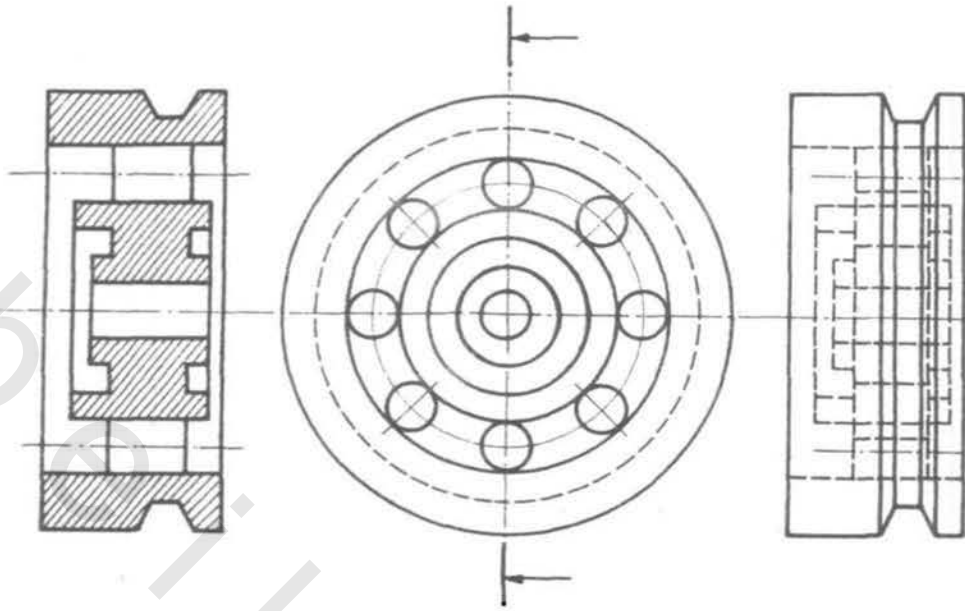
شكل « ١, ٨ » صغوبة فهم المسقط بسبب تزامم الخطوط واستخدام القطع للتوضيح .
