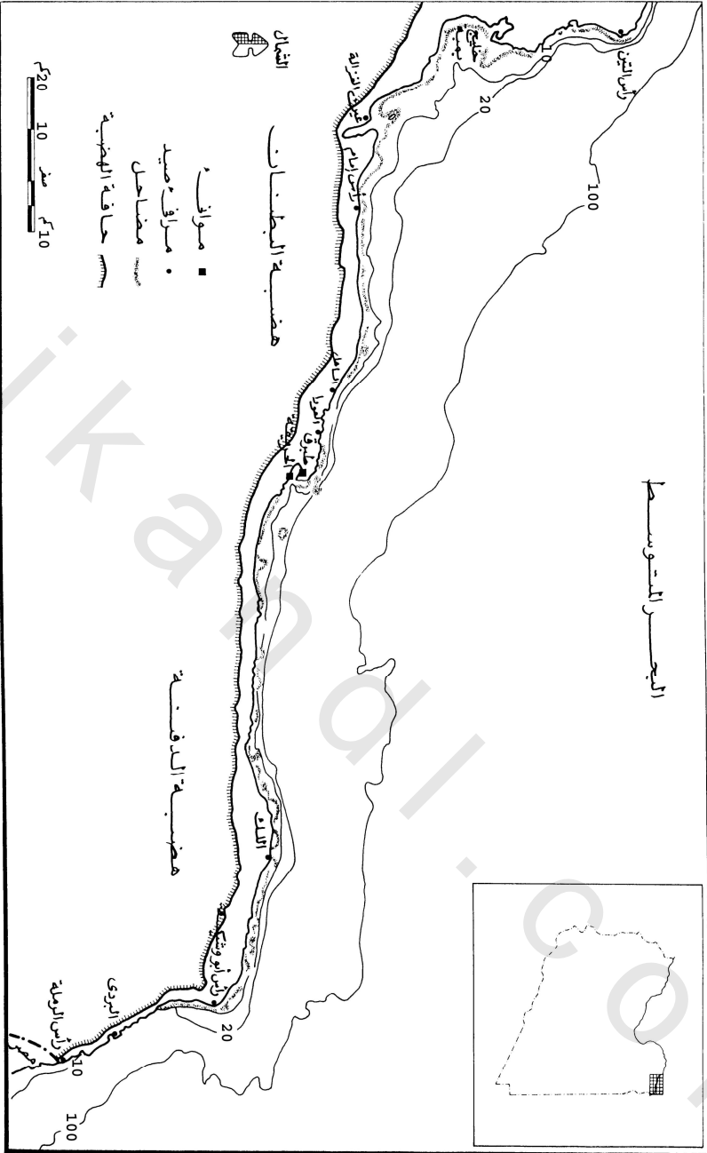
شكل (8-ب) خط الساحل فيما بين شُوكرة ورأس الشوكرة
