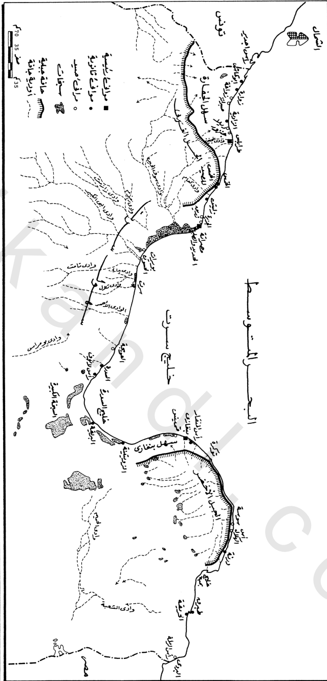
شكل (1) الملامح المورفولوجية للساحل المديني
