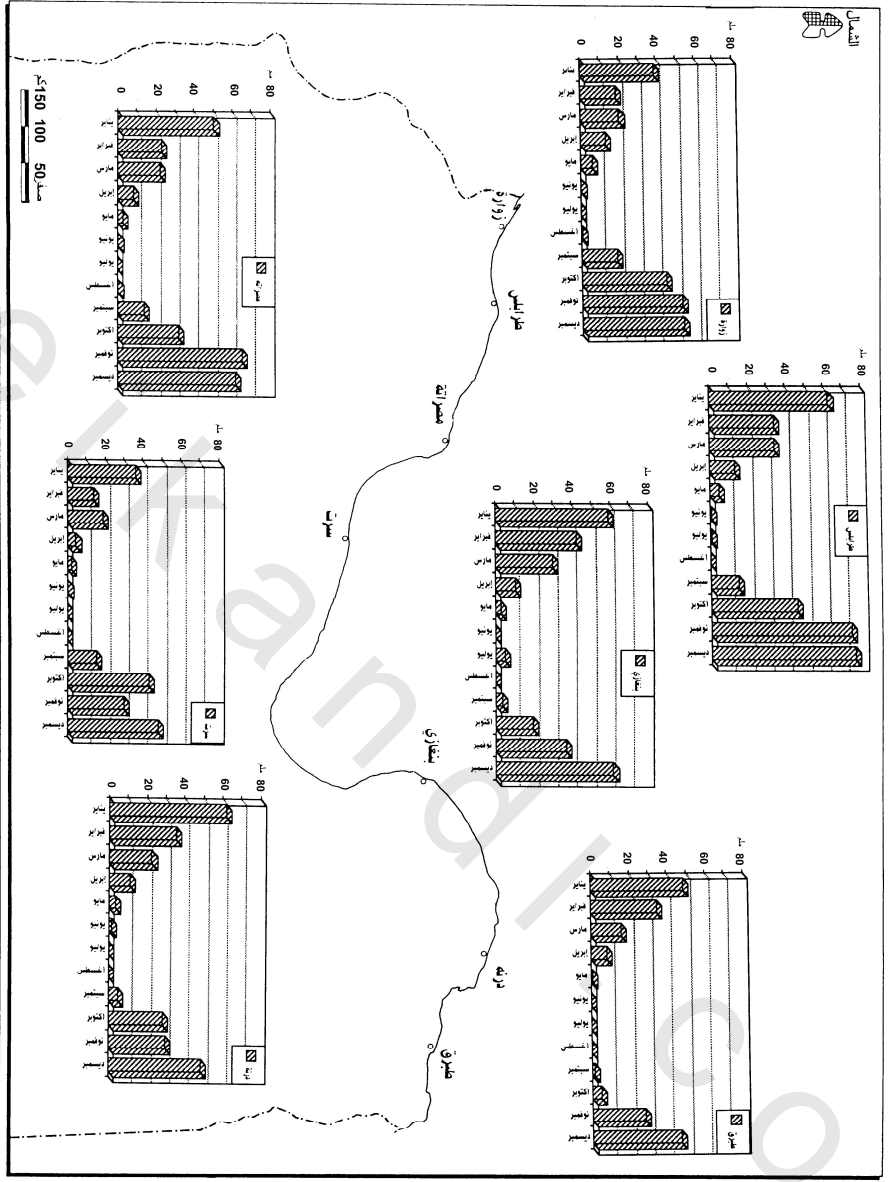
شكل رقم (16) المتوسط السنوي للمطر في محطات الساحل الليبي في الفترة من (1970-1990)
