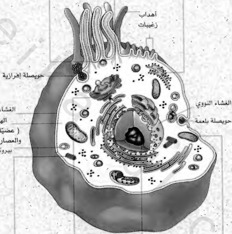
جسيم حال
