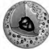
نواة الخلية
