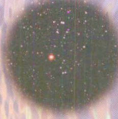
Aldebaran
