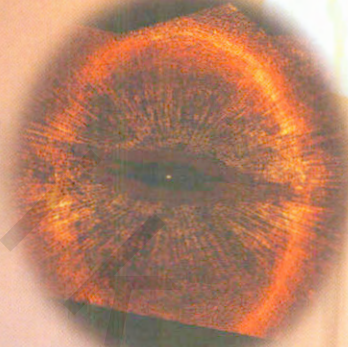
Fomalhaut
