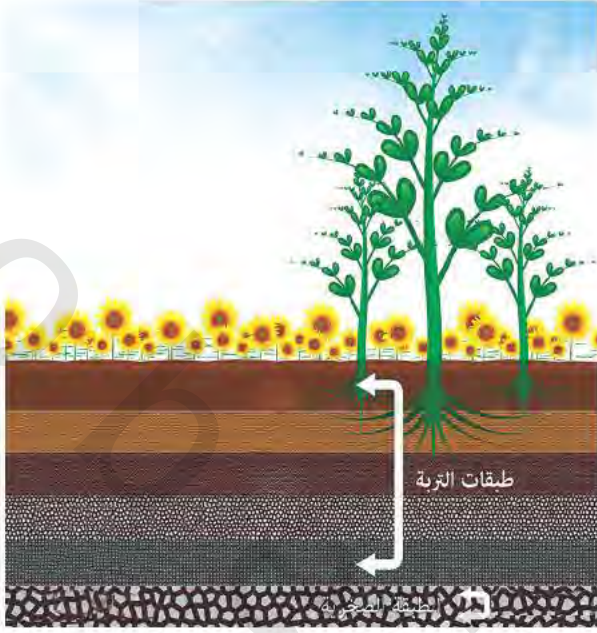
الشكل (١٨-١): رسم تخطيطي لقطاع التربة يوضح نطاقها الأربعة.
