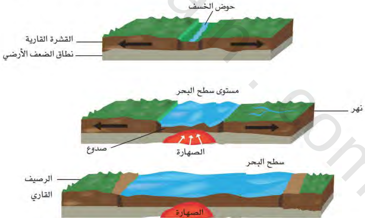
الشكل (٧-١): توسّع قيعان البحار والمحيطات عن طريق تكون الخسوف الأرضية، واندفاعات الصحارة عبرها باستمرار.
