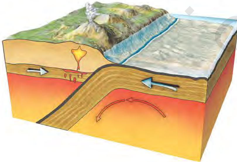
الشكل (١-٥): كيفية تحرك ألواح الغلاف الصخري للأرض.
