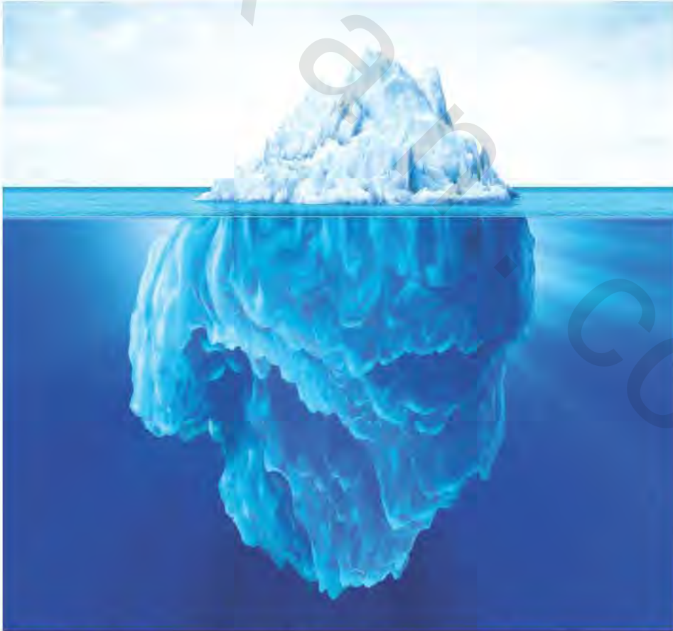
الشكل (٨-٢): جبل من الجليد يعموم في مياه المحيط الأطلسي الجنوبي، وهو يشبه الجبل الصخري في امتداد جذره في الأعماق.
