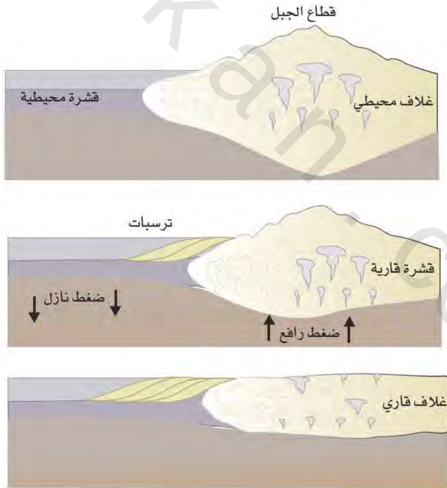
الشكل (٨-١): حركة بروز جذور الجبال كلما برت عوامل التعرية قممها.
