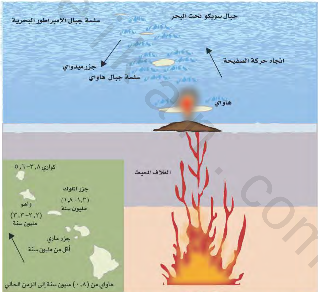
الشكل (٧-٢): رسم تخطيطي لتكوّن الجزر البركانية (مثل جزر هاواي)، بسبب اندفاع الصحارة من نطاق الضعف الأرضي عبر صدوع قيعان المحيطات.
