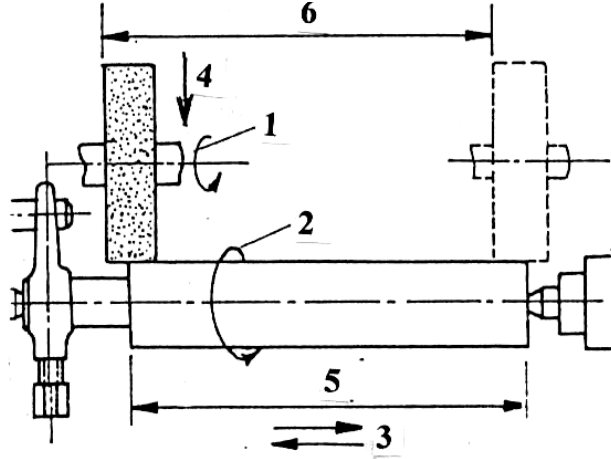
شكل 4 - 25 التجليخ الأسطواني الخارجي
