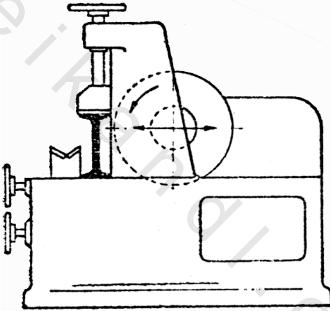
شكل ٢ - ١٧ منشار صينية
