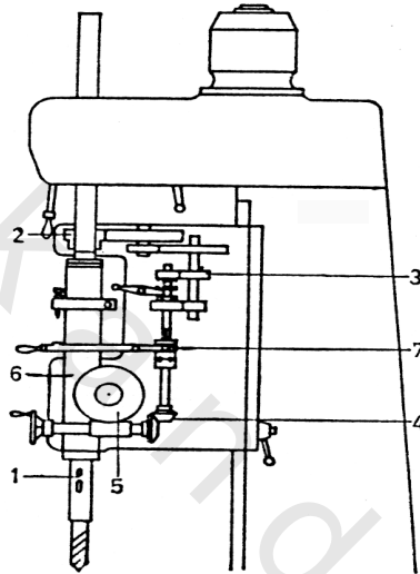
صندوق تروس التغذية بمثقاب قائم
