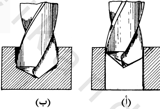
شكل ٣ - ٤ عملية الثقب
