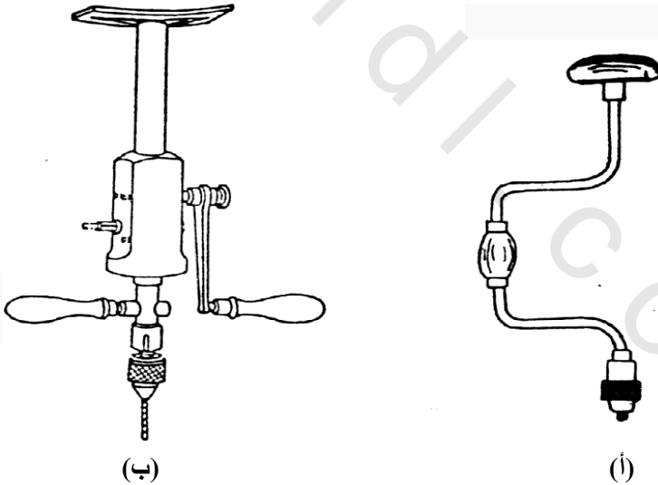
شكل ٣ - ١١ مثقاب يدوي
