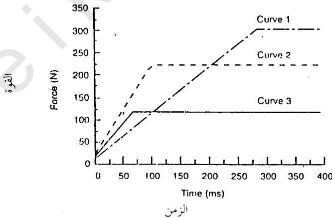
شكل (١) المنحنيات النظرية (القوة-الزمن) لأفراد مختلفين فى مستوى القدرة
