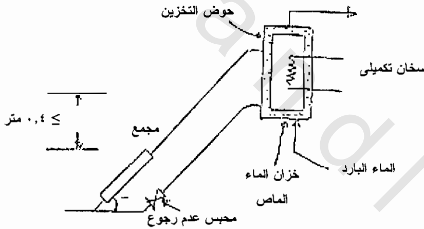
شكل (٣/١) مخطط لسخان الماء الشمسى بالتدوير الطبيعى مع إضافة طاقة إلى حوض التخزين (مضغوط)
