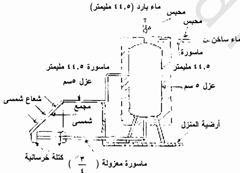
شكل (٣/٢ - ب) سخان الماء الشمسى التقليدى
