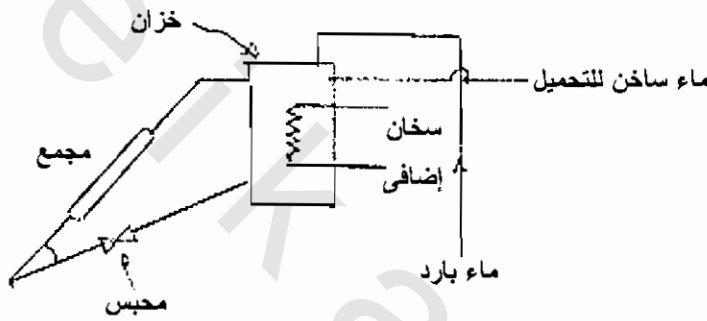
شكل (٣/٢ - أ) سخان الماء الشمسى بدون ضغط
