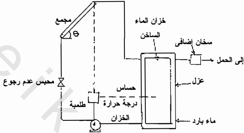
شكل (٣/٣) مخطط للتدوير عنوة لسخان الماء الشمسى مع الحمل الإضافى على الخط
