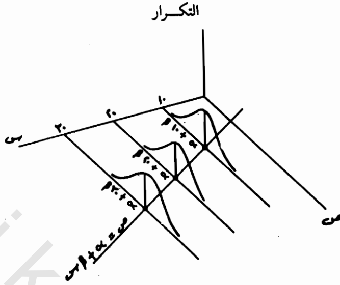
الشكل (٩ - ٤) توزيعات معدلة للمتغير ص عند s = ١٠, ٢٠, ٣٠
