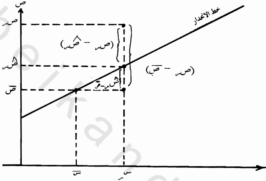
الشكل (٩ - ٥) : تجزئة الاختلاف فى المتغير ص
