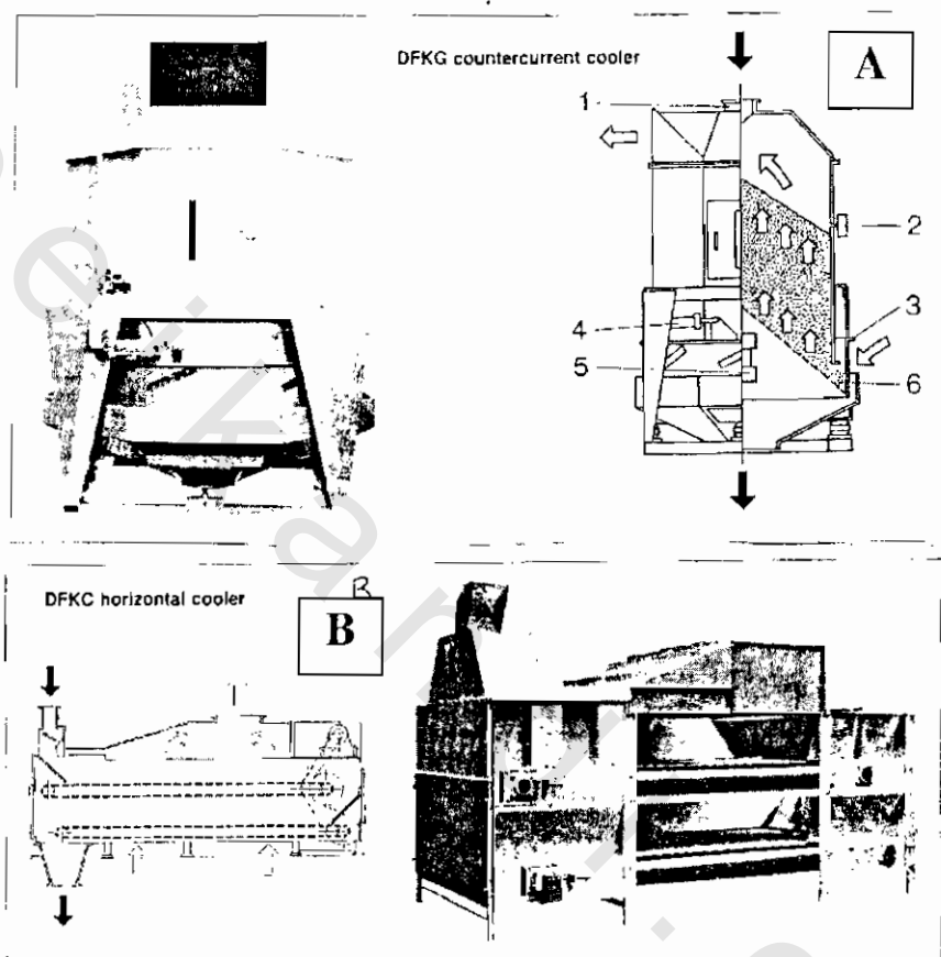
شكل رقم ( ١٦ - ٢ ) وحدة تبريد منتجات مصنعة رأسية ( A ) شكل رقم ( ١٦ - ٣ ) وحدة تبريد منتجات مصنعة أفقية ( B ) اختلاف في تصميم الأجهزة
