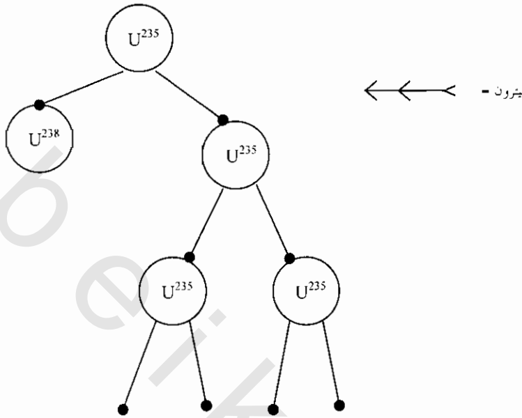
شكل رقم (١): الانشطار النووي لليورانيوم ٢٣٥
