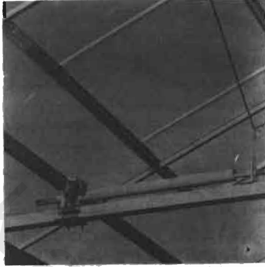
شكل ( ٣ - ٢٨ ) : نظام التحكم الآلى فى فتحات التهوية ( عن J.t.provence - فرنسا ) .
