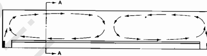
قطاع طولى
