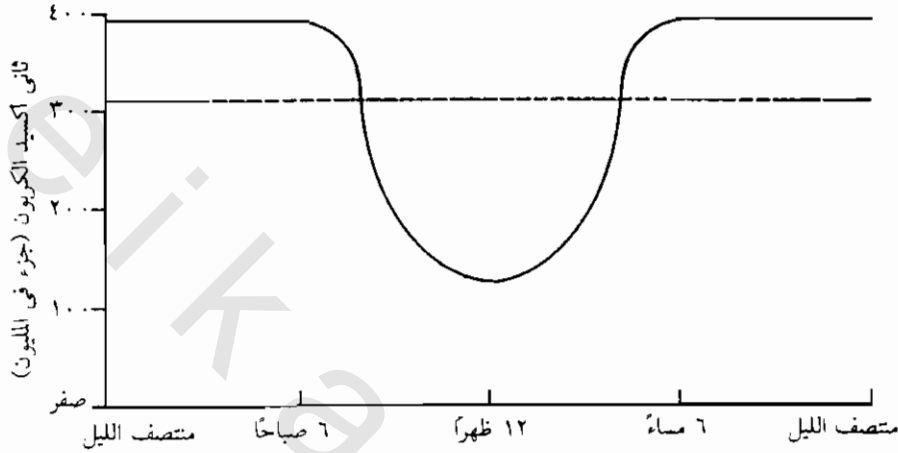
شكل ( ٣ - ٣٦ ) : التغيرات فى نسبة غاز ثاني أكسيد الكربون فى البيوت المحمية المغلقة ( الخط البياني المتصل ) ، مقارنة بنسبة الغاز فى الهواء الطلق ( الخط المنقطع ) ( عن Ball ١٩٨٥ )
