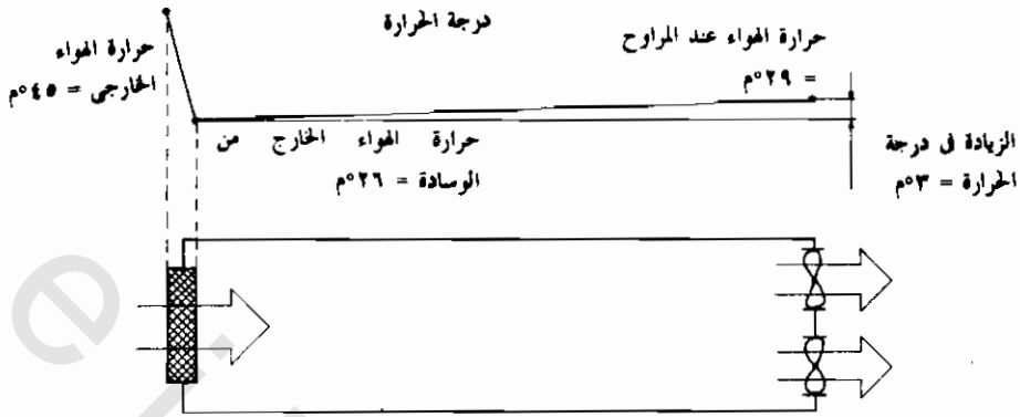
شكل ( ٣ - ٩ ) : التغيرات فى درجة حرارة الهواء الخارج خلال البيوت المبردة بنظام المروحة والوسادة .
