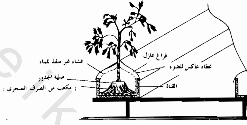
شكل ( ٦ - ٣ ) : قناة تقنية الغشاء المغذى ، وقد بظنت بالبولىثيلين .
