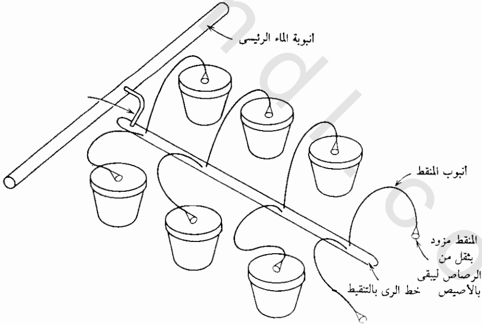
شكل ( ٥ - ٧ ) : ري نباتات الأصص بالتنقيط .
