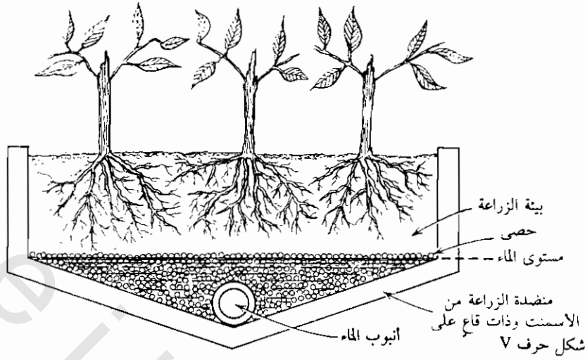
شكل (٦-٧) : رى النباتات النامية فى مناضد الزراعة ( البنشات ) بطريقة الرى تحت السطحى .
