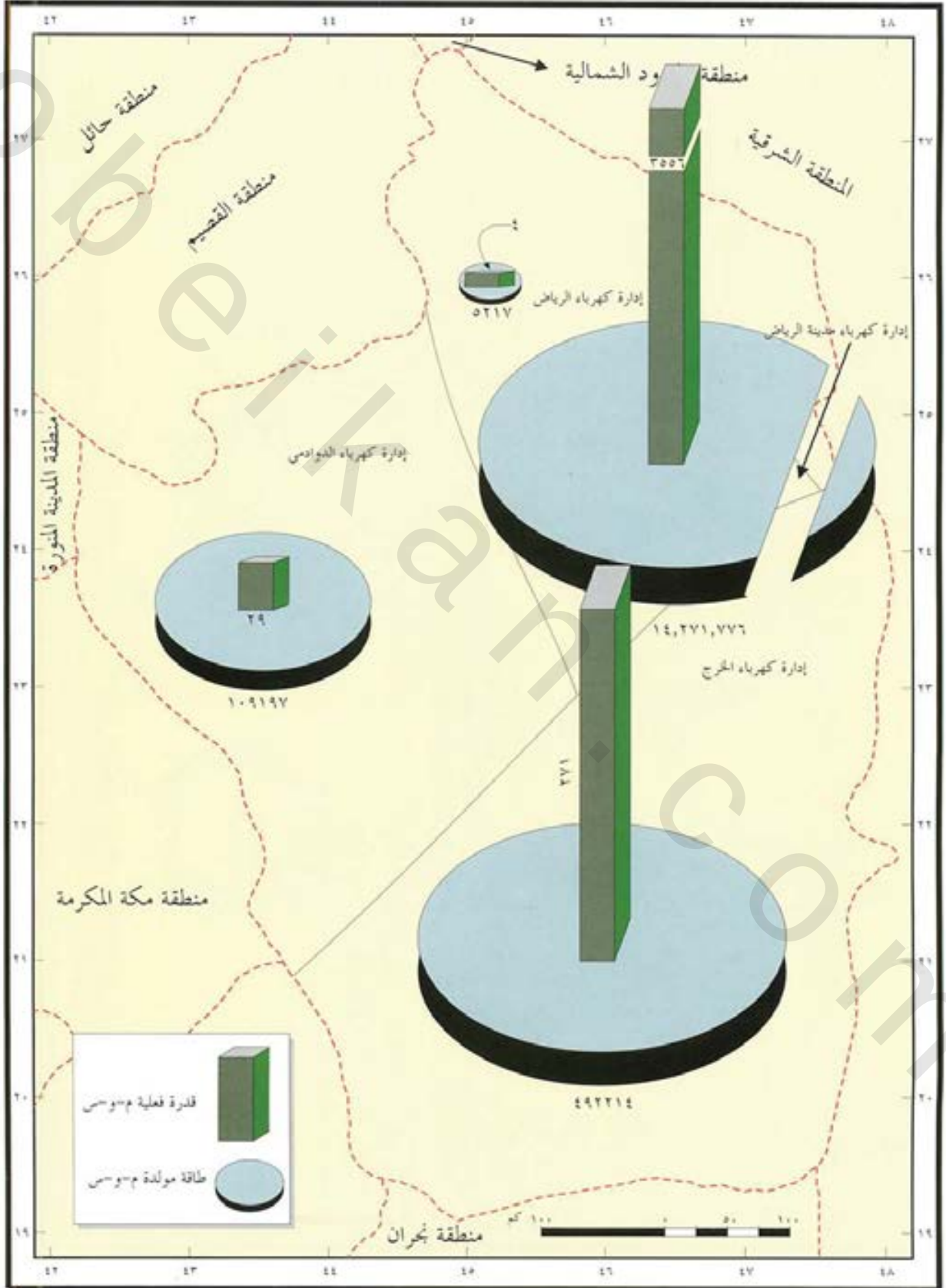
شكل (٧-٣-٢) توزيع القدرات الفعلية والطاقة المولدة في منطقة الرياض لعام ١٤١٧هـ
