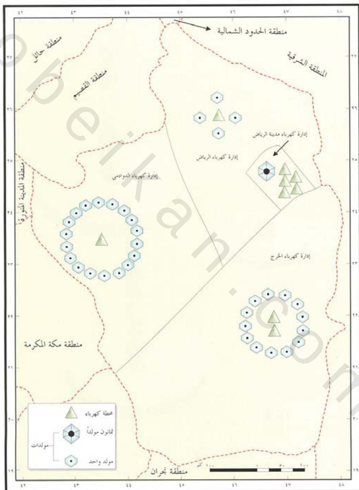
شكل (٧-٣-١) توزيع عدد المحطات والمولدات الكهربائية في منطقة الرياض لعام ١٤١٧هـ
