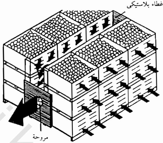
شكل ( ١٣ - ١ ) : مسار الهواء في التبريد الآلي بطريقة السريان الجبري للهواء ( عن Wills وآخرين ١٩٨١ ) .
