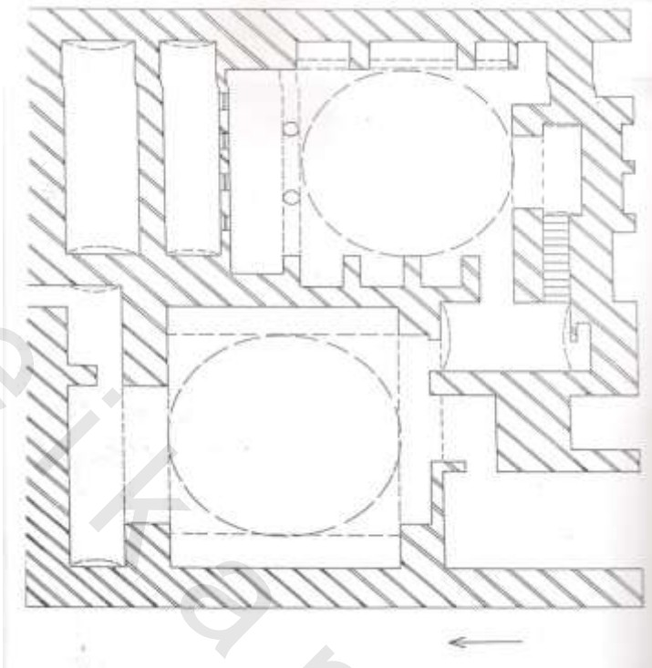
مخطط (١) مخطط ارضي لحمام سعيد الشروفي
