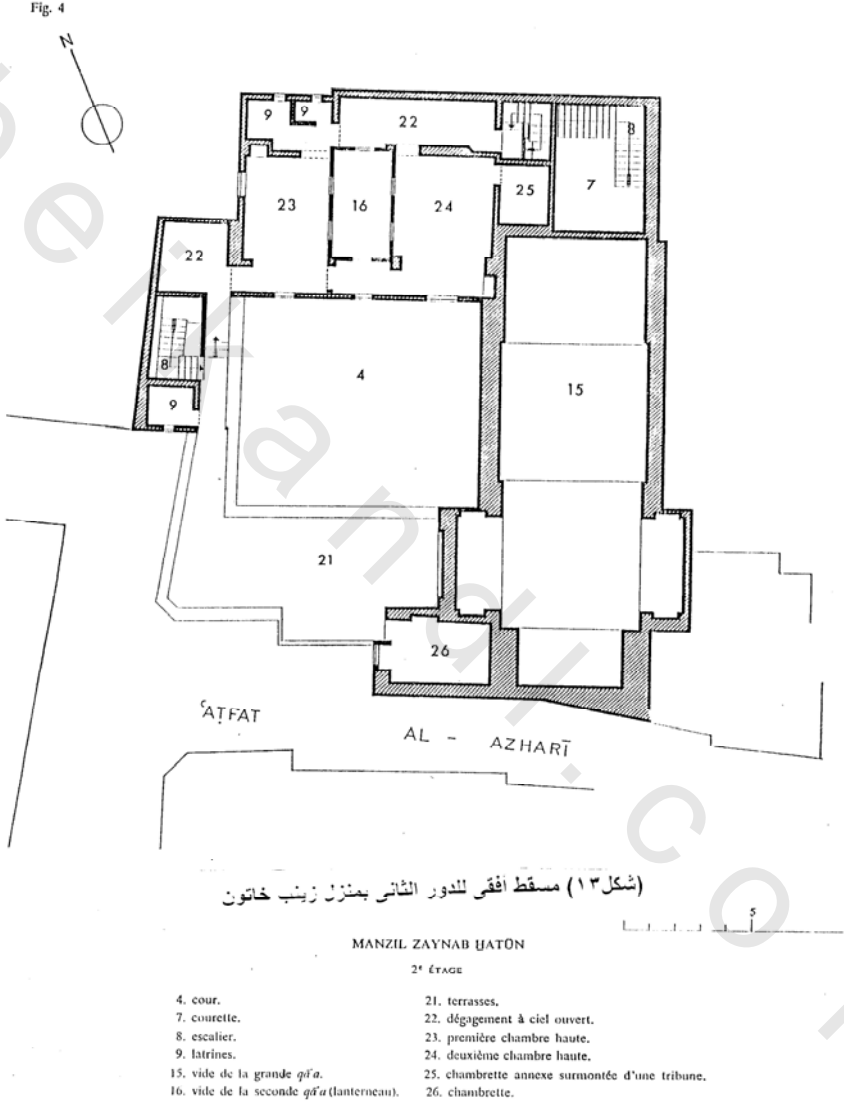
(شكل 13) مسقط أفقي للدور الثاني بمنزل زينب خاتون
