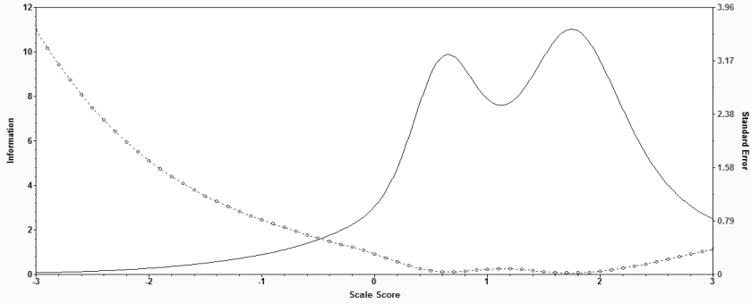
شكل (٣) : دالة معلومات الاختبار للنموذج الثالث للاختبار والخطأ المعياري للقياس
