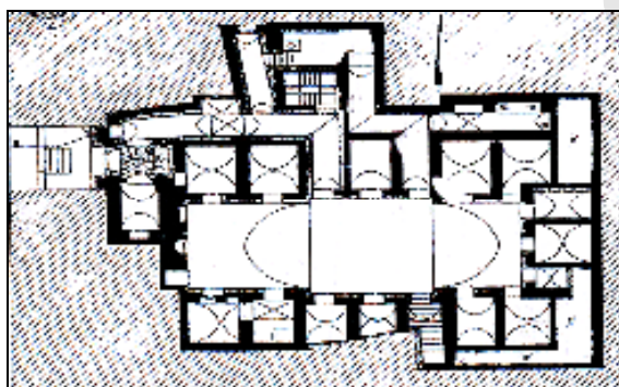
شكل ٦ - المسقط الأفقي لرباط زوجة إينال عن المجلس الأعلى للآثار
